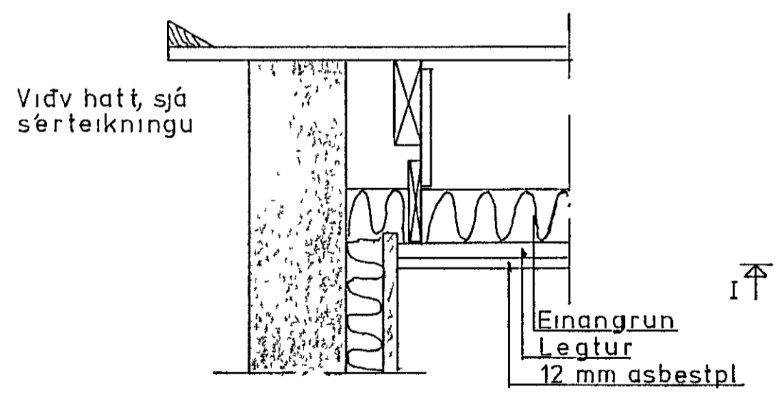
SNID I-I mál 1:10 þak í kyndingu
