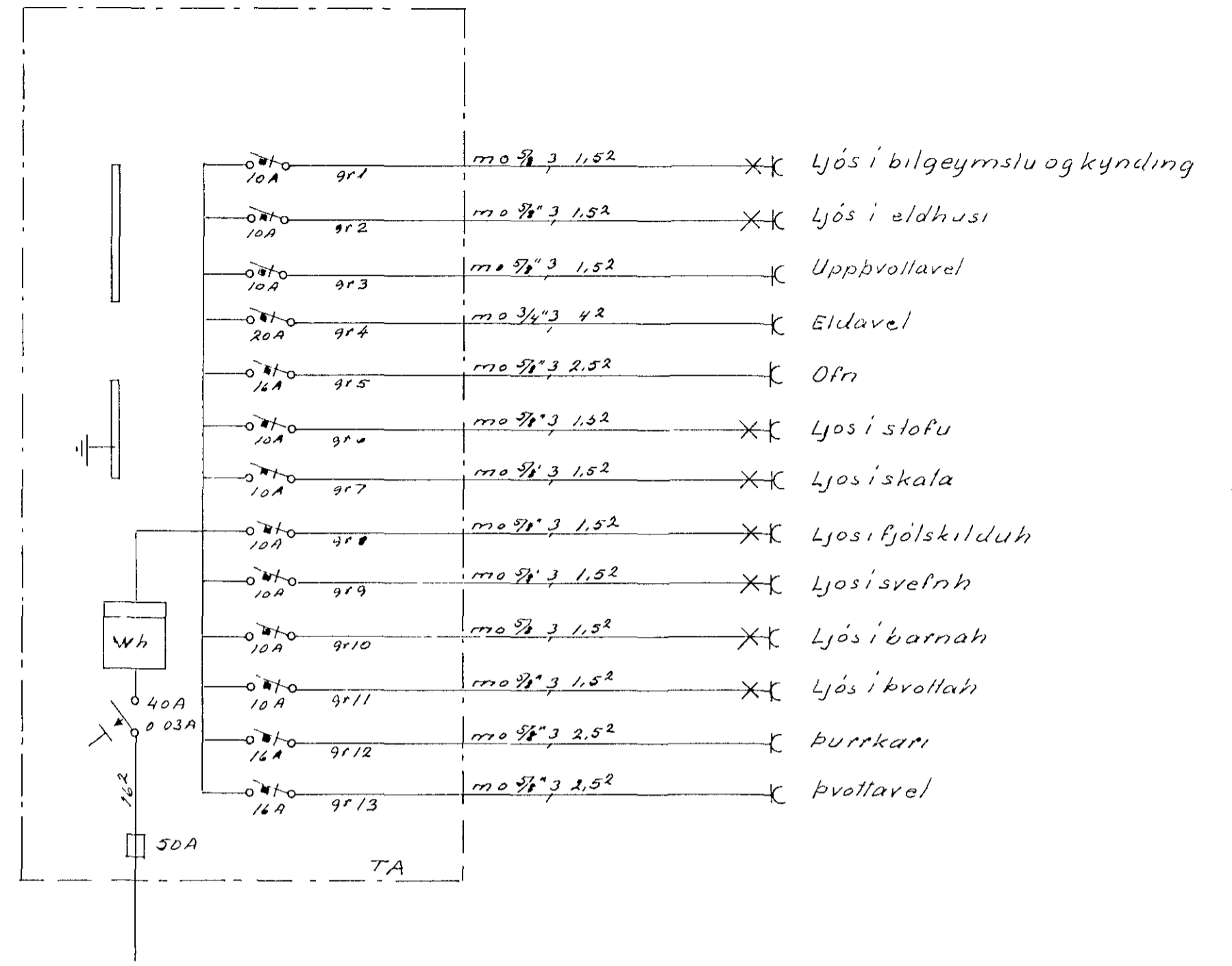
EINLÍNUMYND AF RAFTÓFLU
