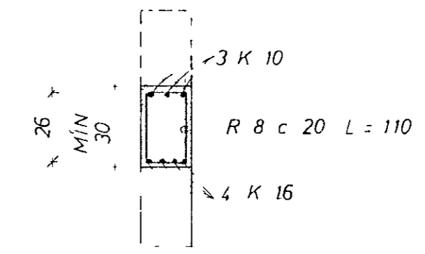
SNID E 1:20
