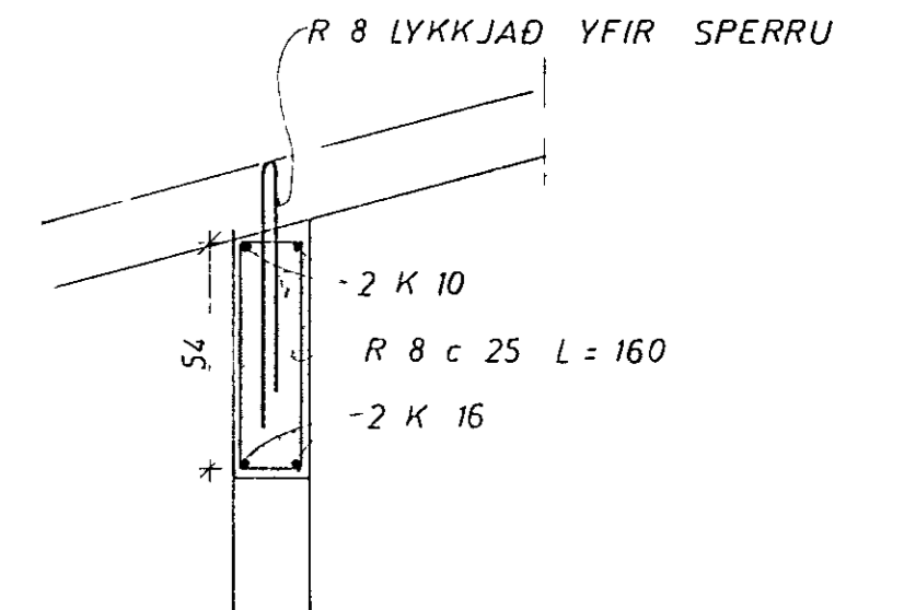
SNID D 1:20
