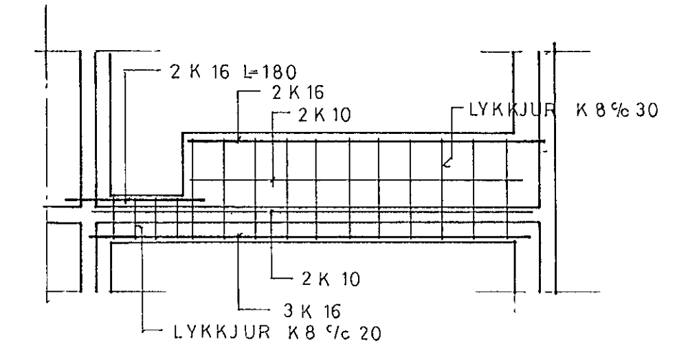
SNID A 150 (A EINNIG VID UM SNID B)
