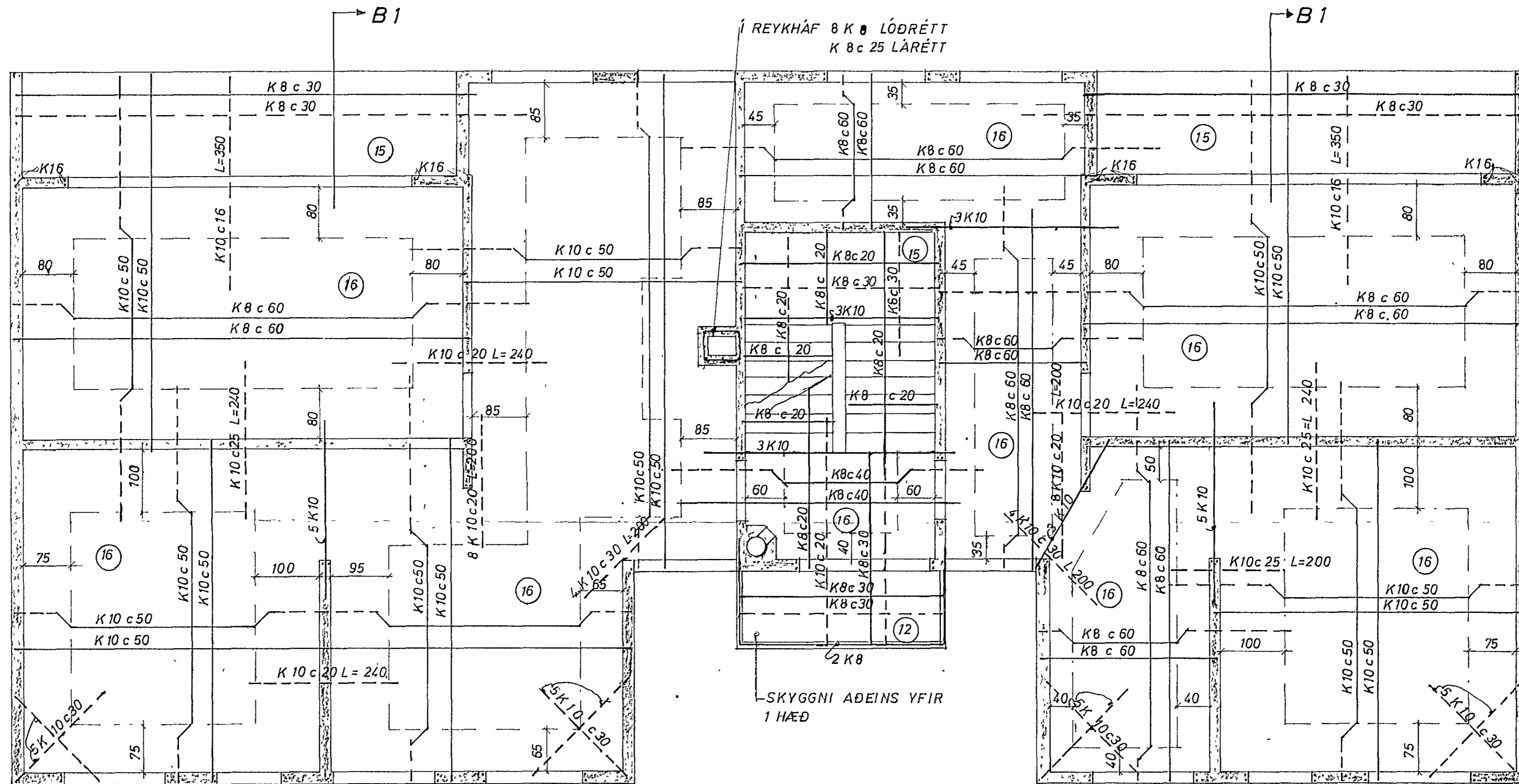
GRUNNMYND 1:50
