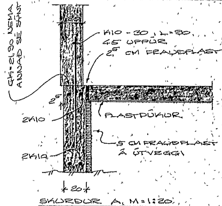
SKURÐUR A, M=1:20
