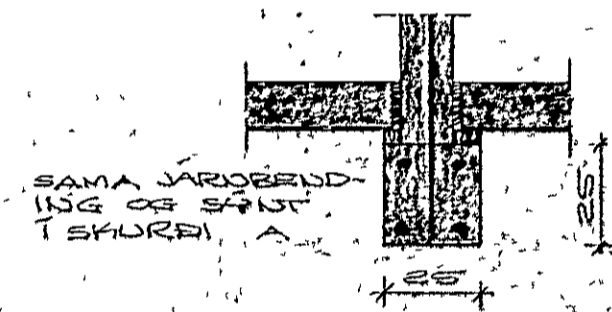
SKURÐUR B, M=1:20
