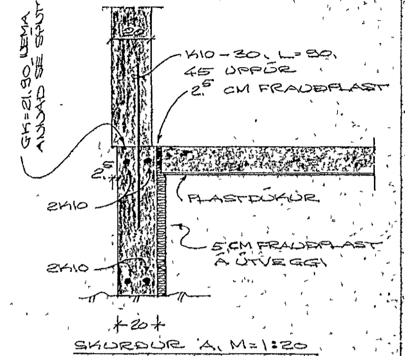
SKURÐUR A, M=1:20
