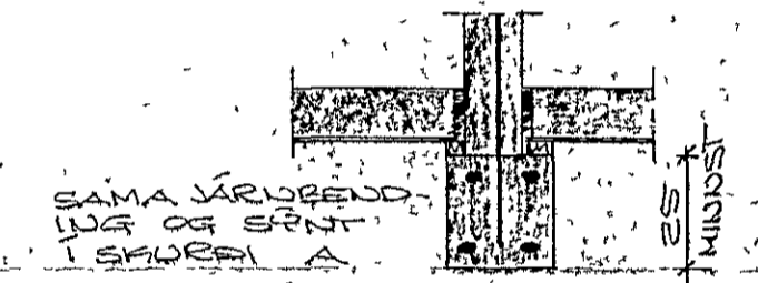
SKURÐUR B, M=1:20
