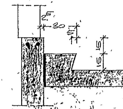
SKURÐUR D, M=1:20
