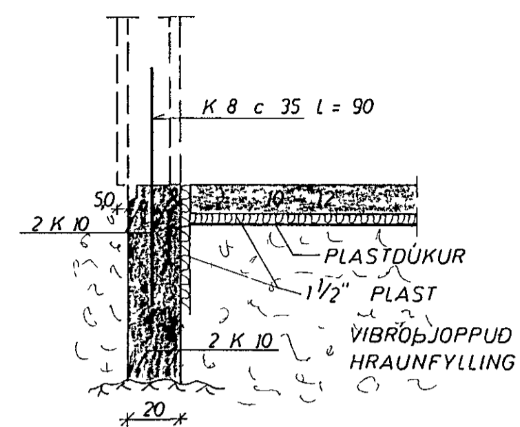
SNID 1 ÚTVEGG 1: 20
