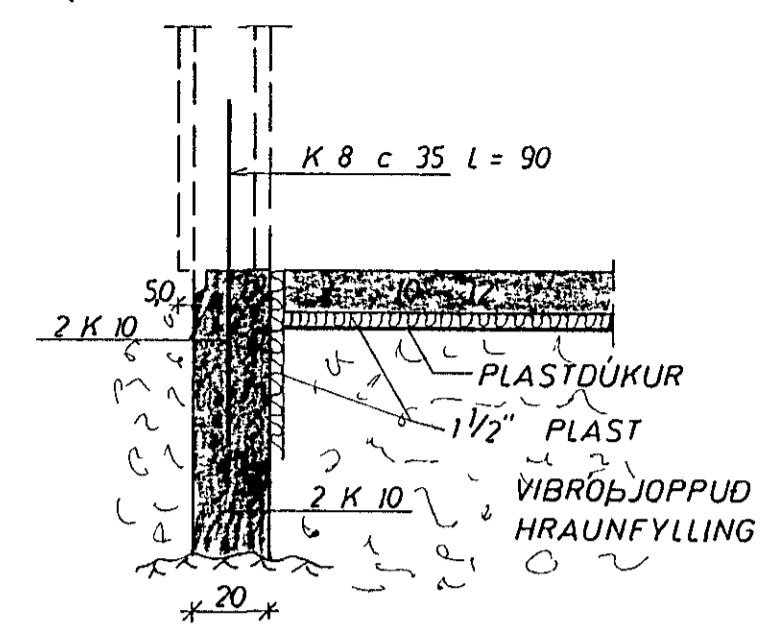
SNID 'I UTVEGG 1: 20
