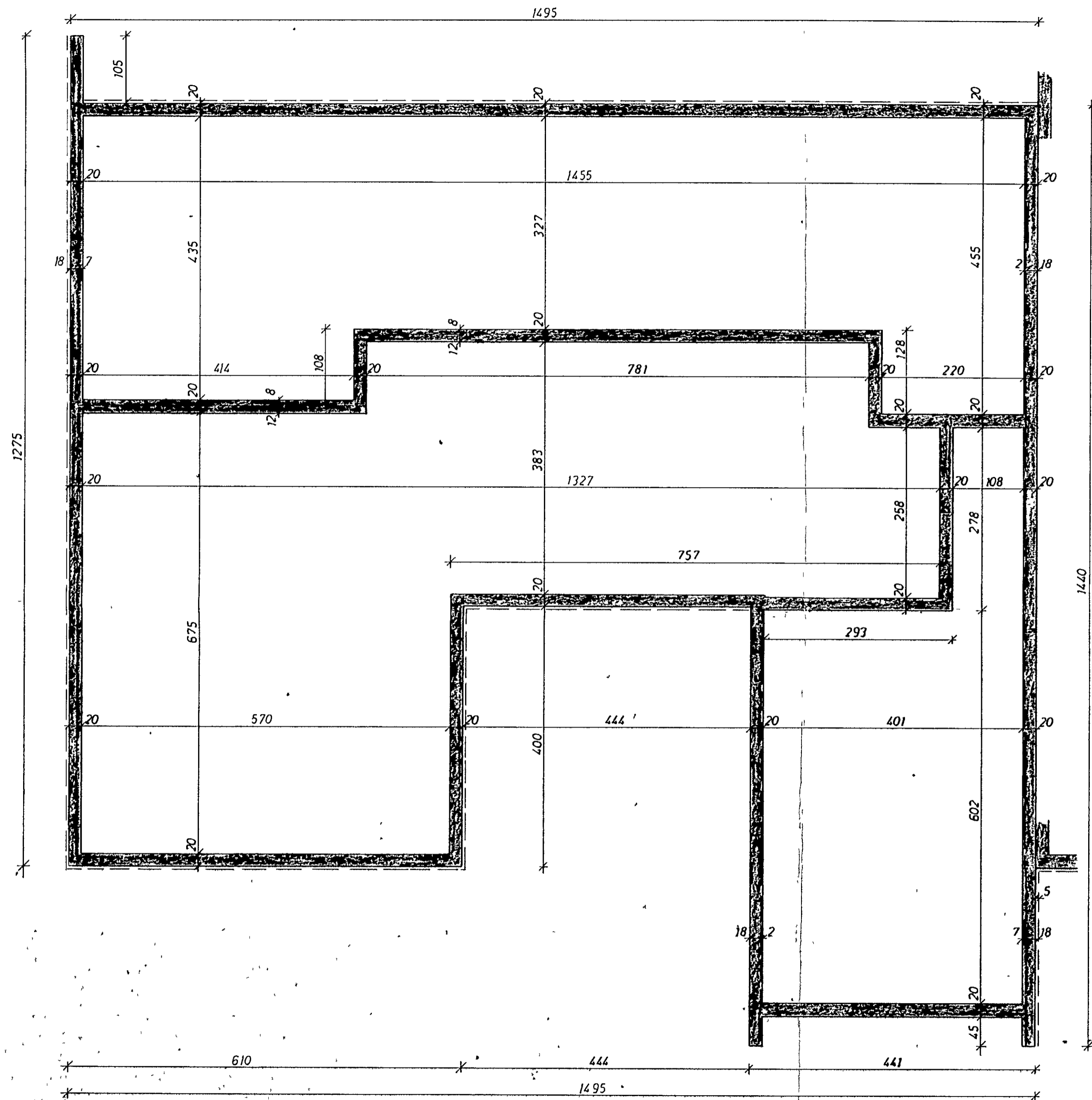
GRUNNMYND 1: 50
