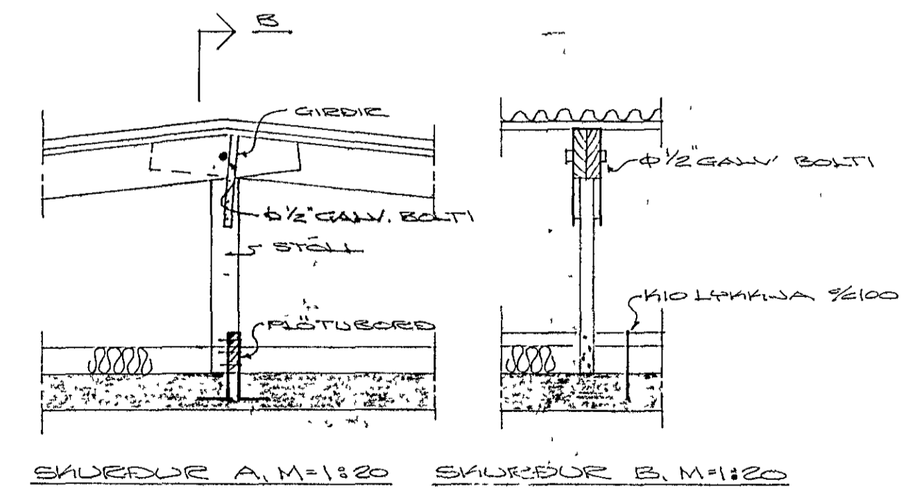
SKURÐUR A, M=1:20 SKURÐUR B, M=1:20
