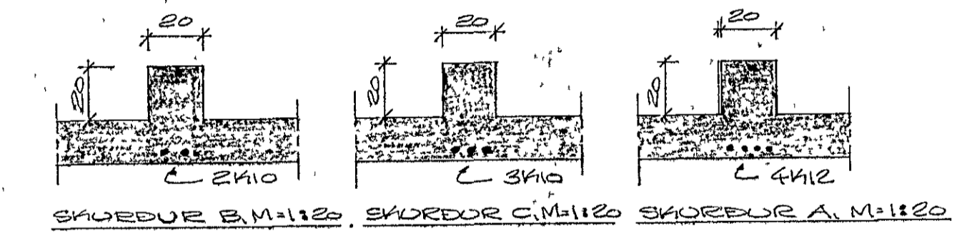
SKJEDUR B, M:1:20 SKJEDUR C, M:1:20 SKJEDUR A, M:1:20
