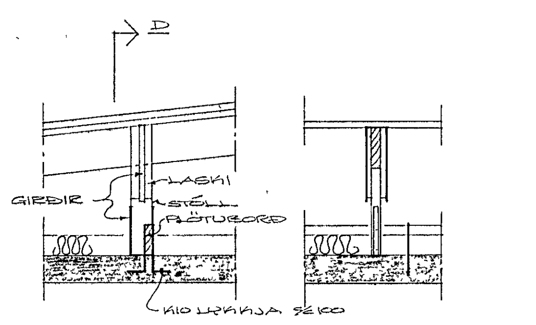
SKURÐUR C, M=1:20 SKURÐUR D, M=1:20
