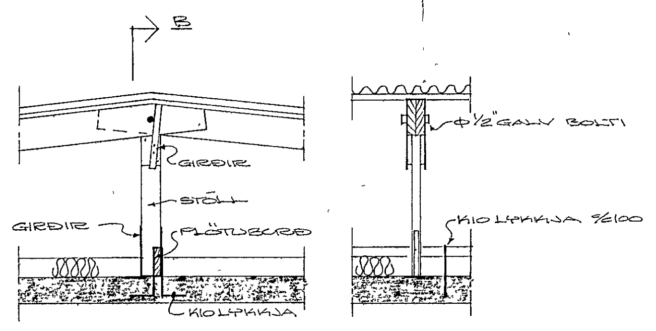
SKURÐUR A, M=1:20 SKURÐUR B, M=1:20
