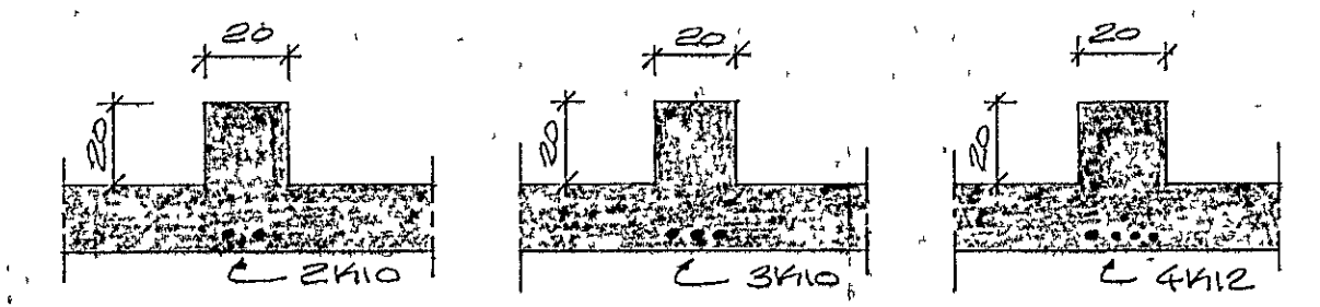
SKURÐUR B, M:1:20 SKURÐUR C, M:1:20 SKURÐUR A, M:1:20
