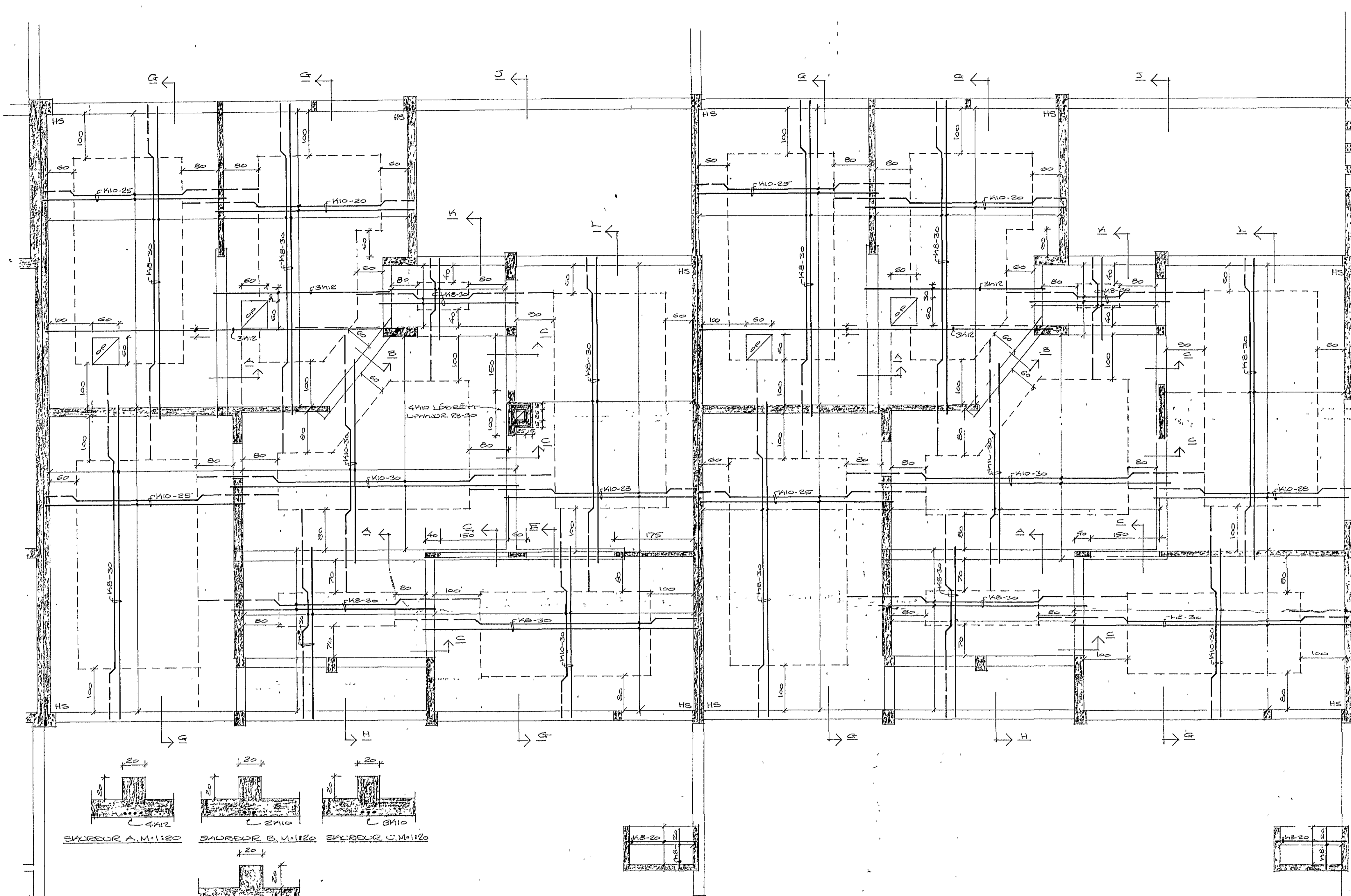
GRÖNDUMFUND, M=1:50
