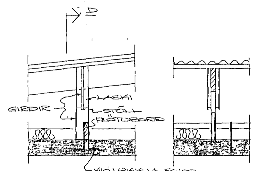
SKURÐUR C, M:1:20 SKURÐUR D, M:1:20
