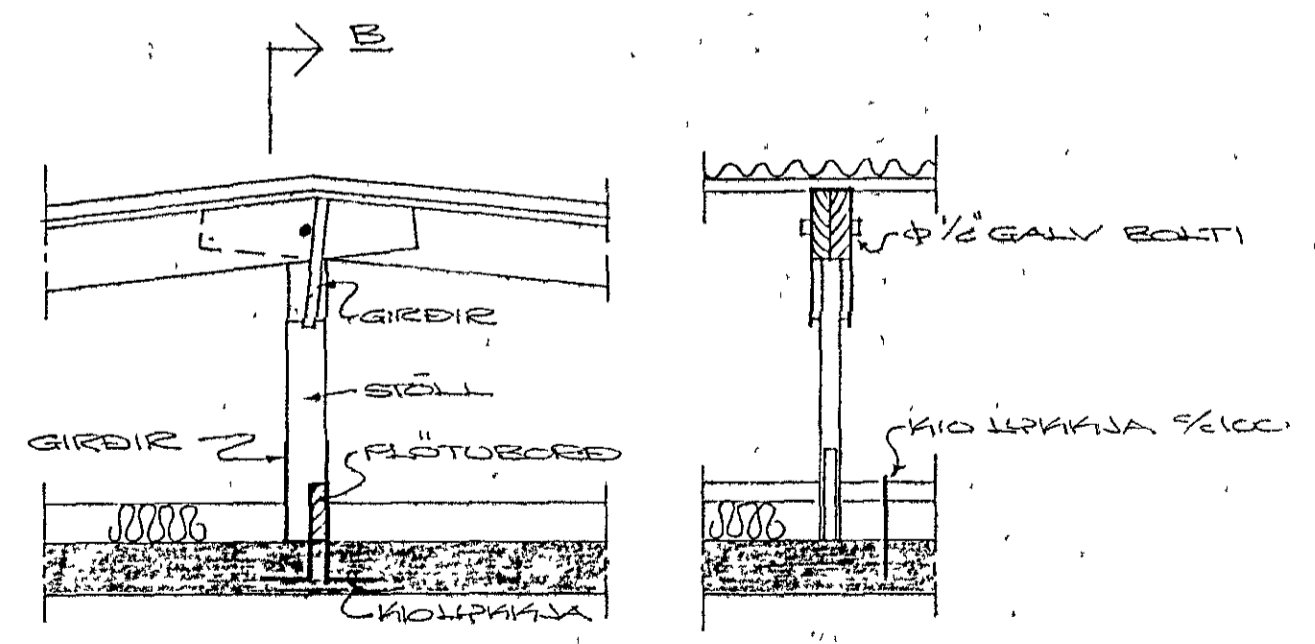
SKURÐUR A, M:1:20 SKURÐUR B, M:1:20
