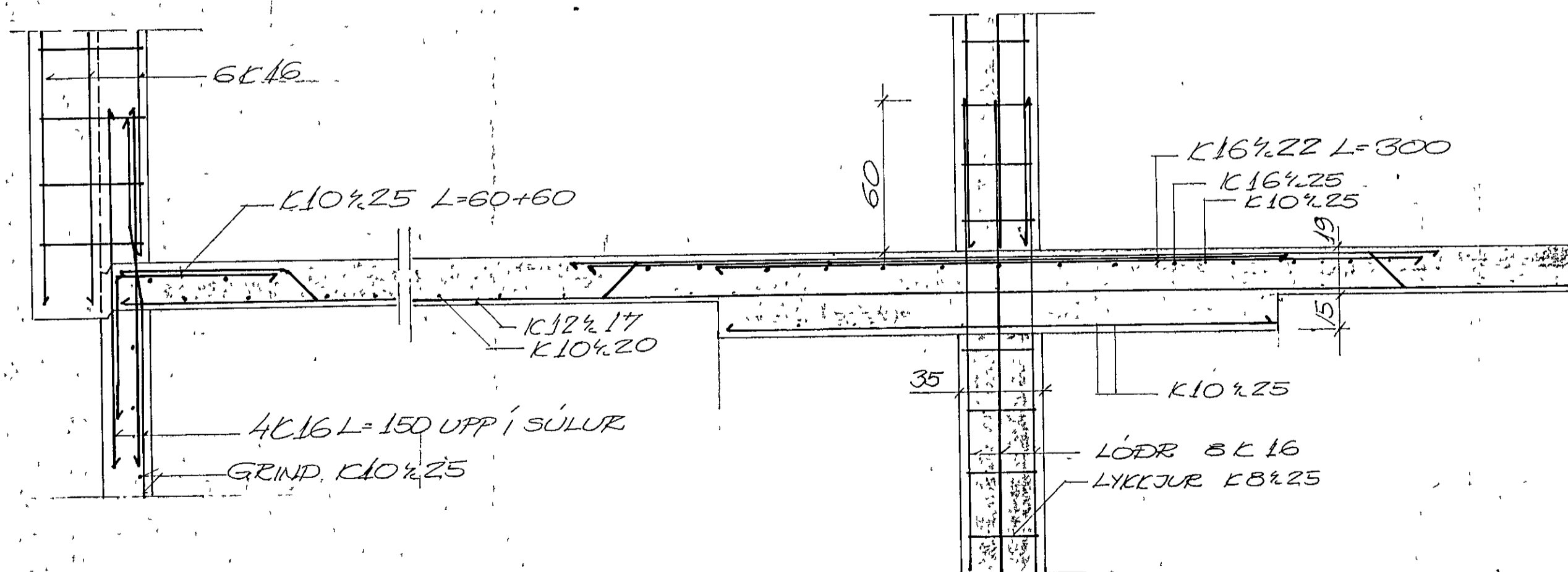
SNID A-A 1:20
