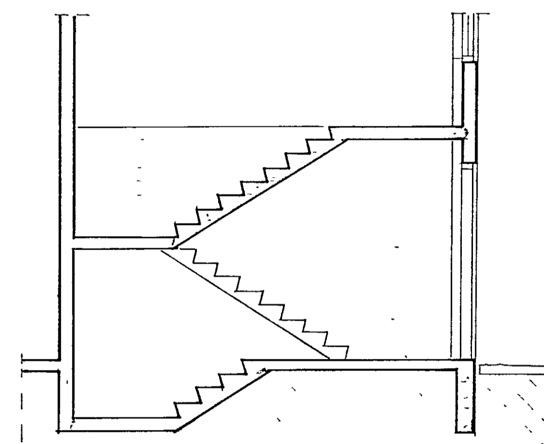
SNEIÐING Í STIGAHÚS 1:50
