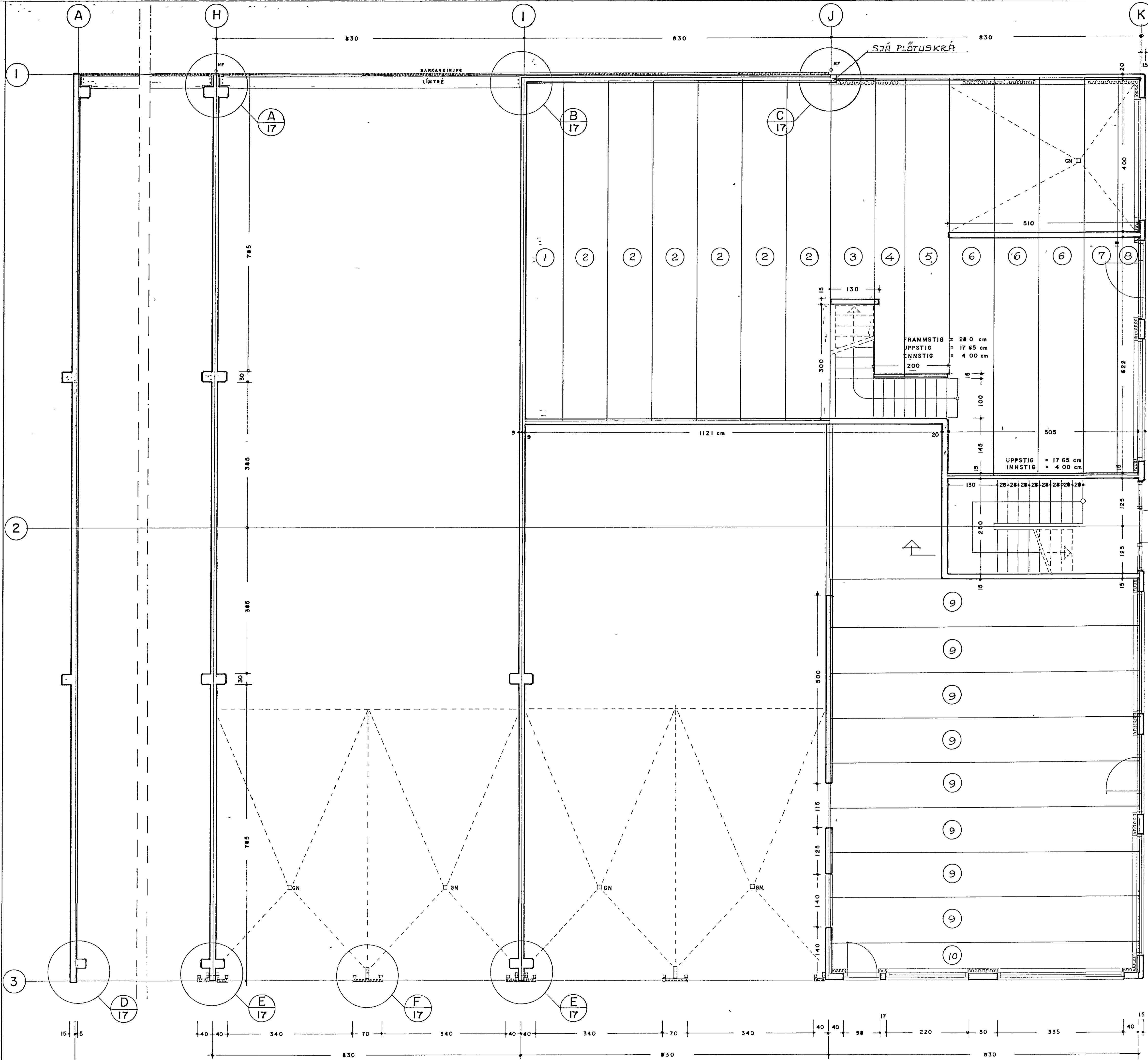
GRUNNMYND JARÐHÆÐ HLOTAMYND. 1:50
