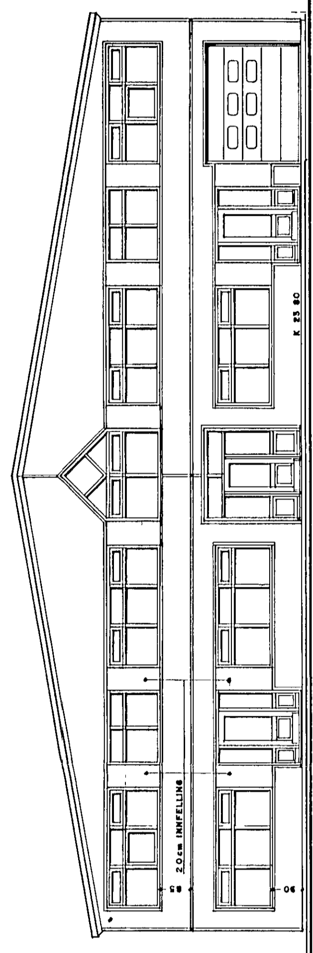
NORÐURHLID. 1:100
