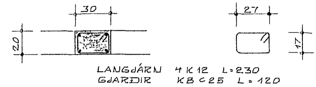
SÚLA S12 1:20
