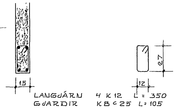
SÚLA S13 1:20
