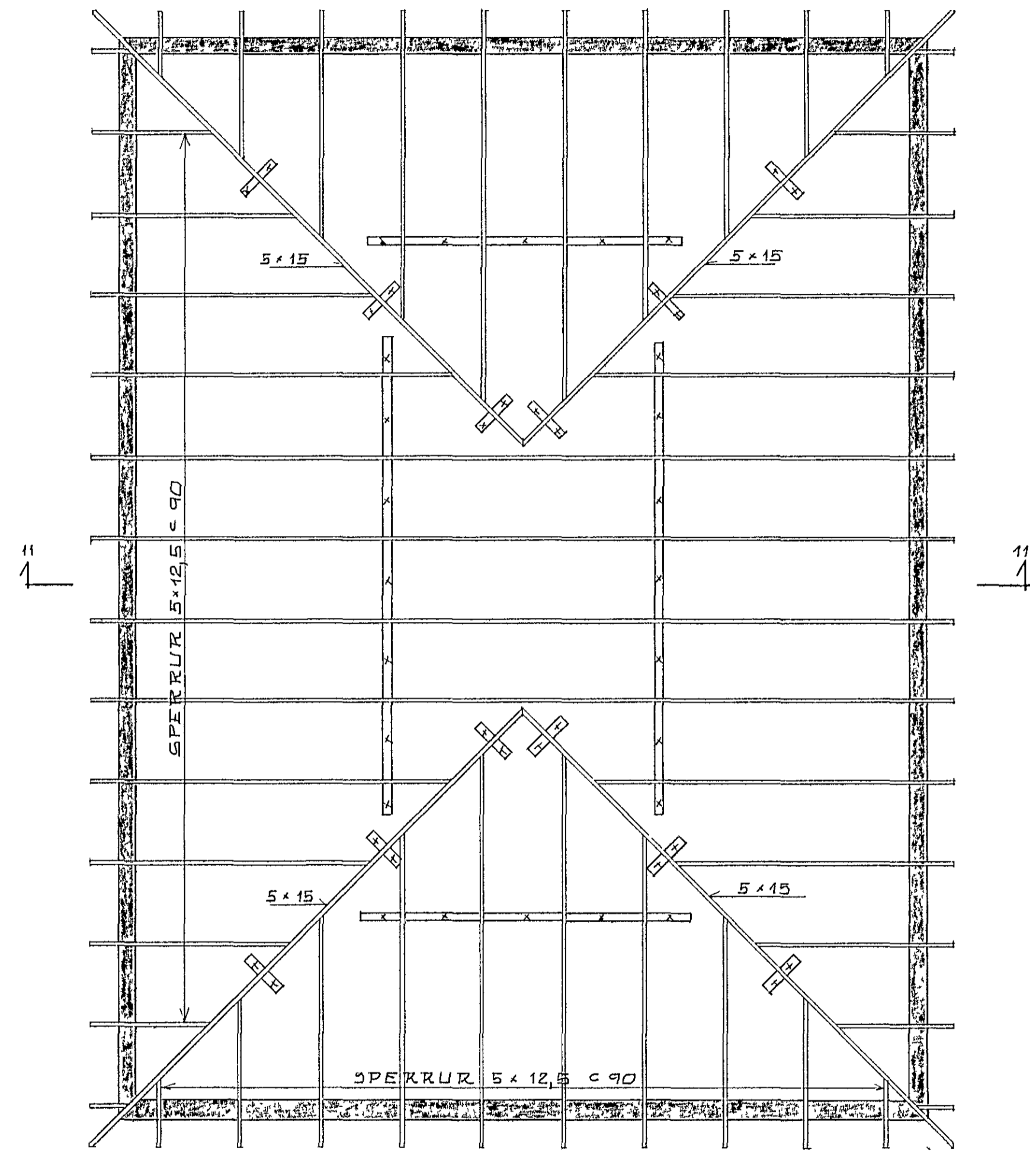
GRUNNMYND 1 50
