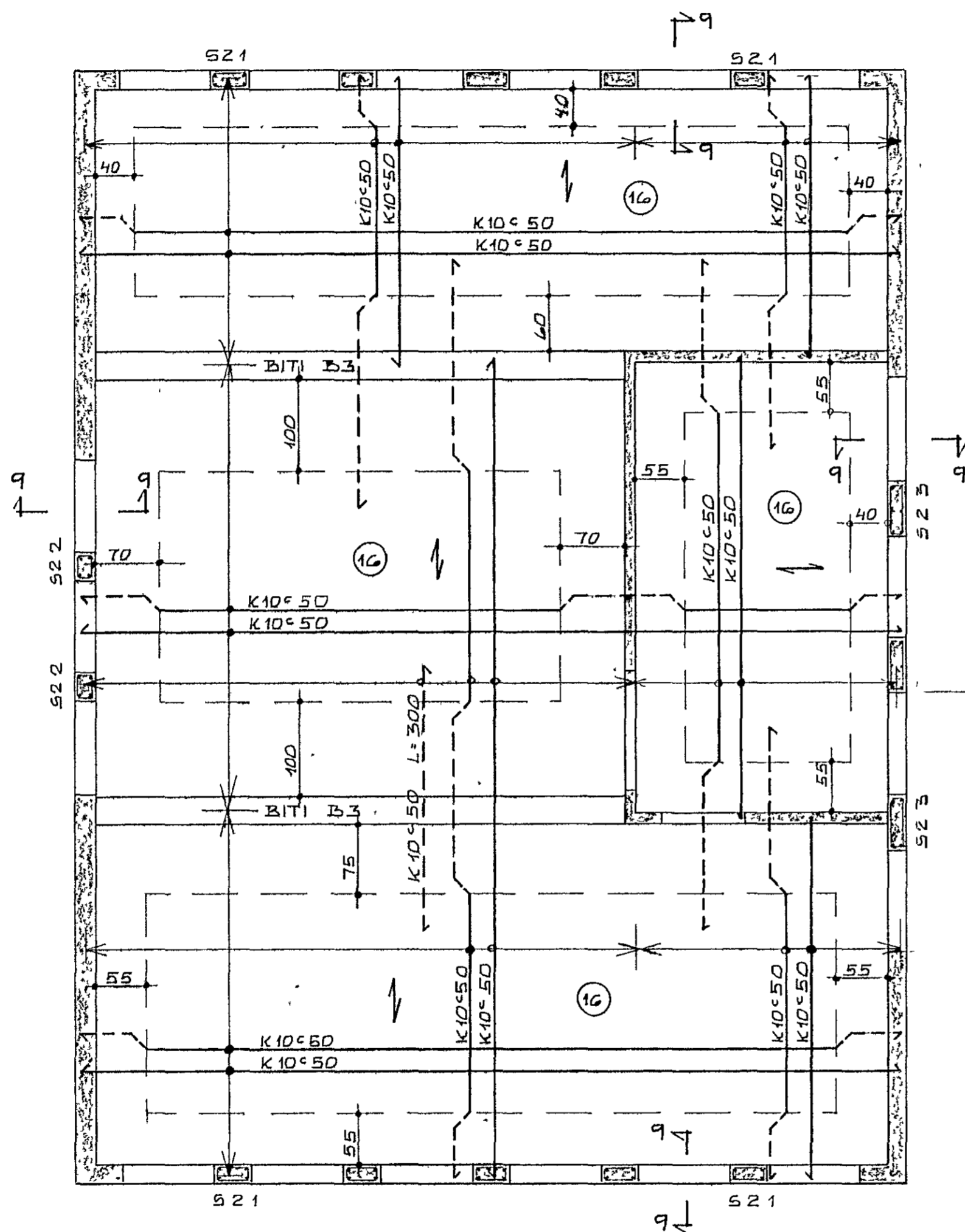
GRUNNMYND 1.50
