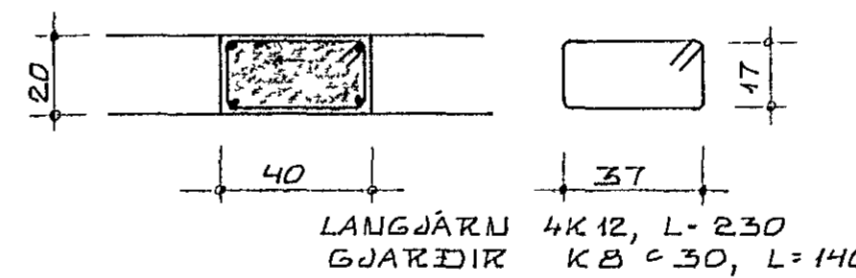
SÚLA S21 1.20
