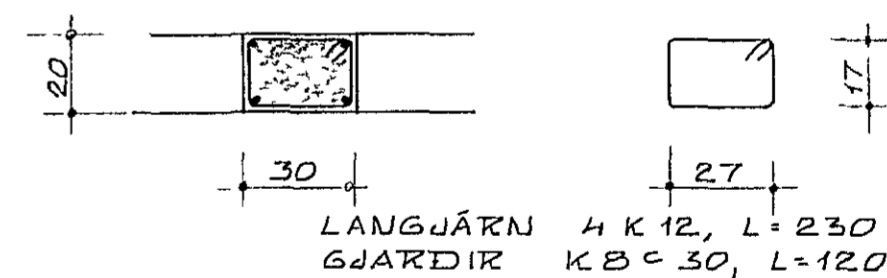
SÚLA S22 1.20
