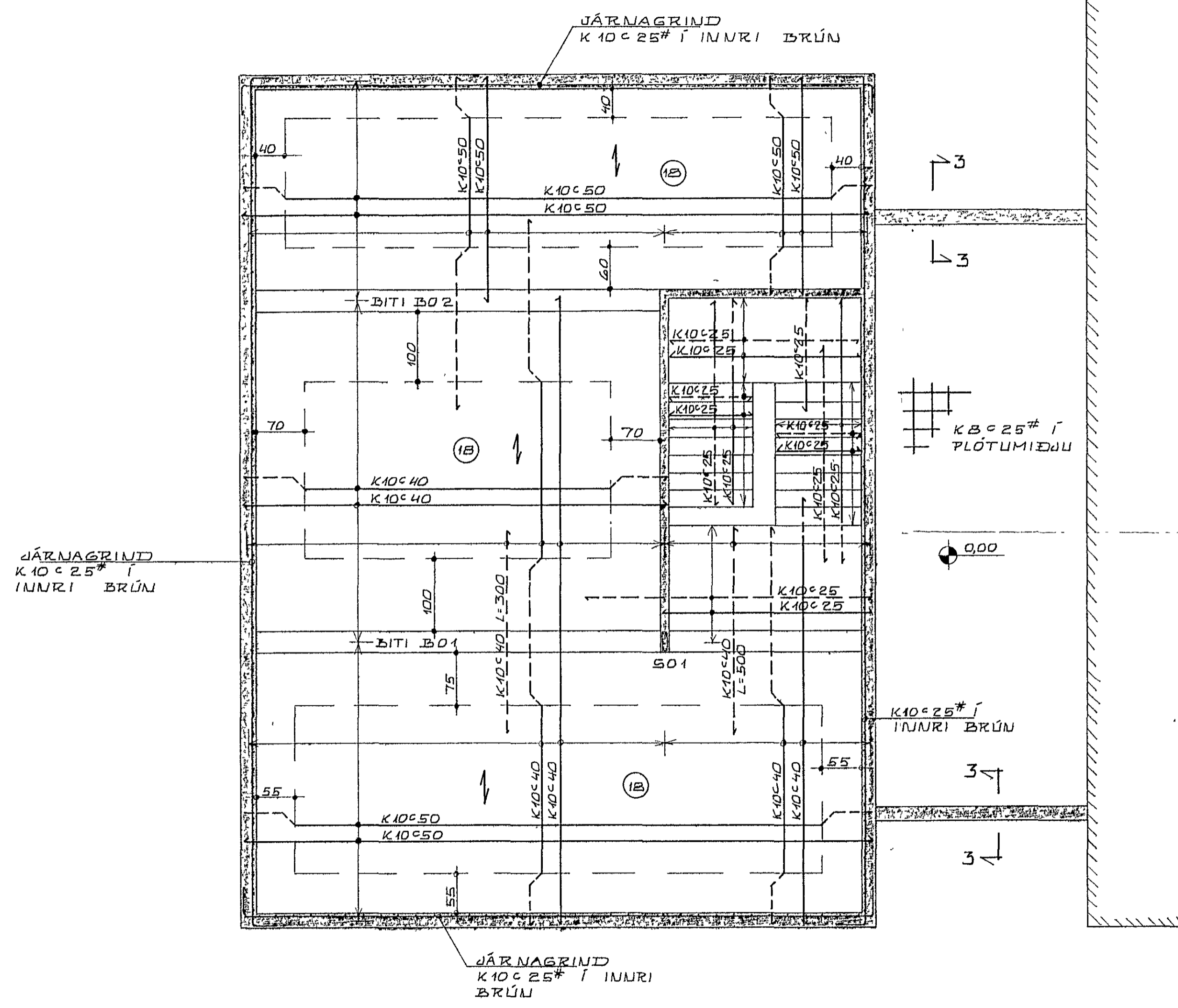
GRUNNMYND 1:50
