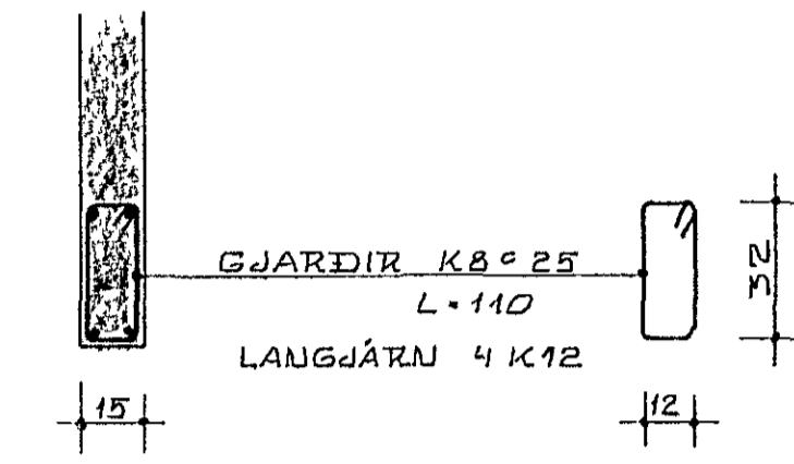
SÚLA S.O.1 1:20
