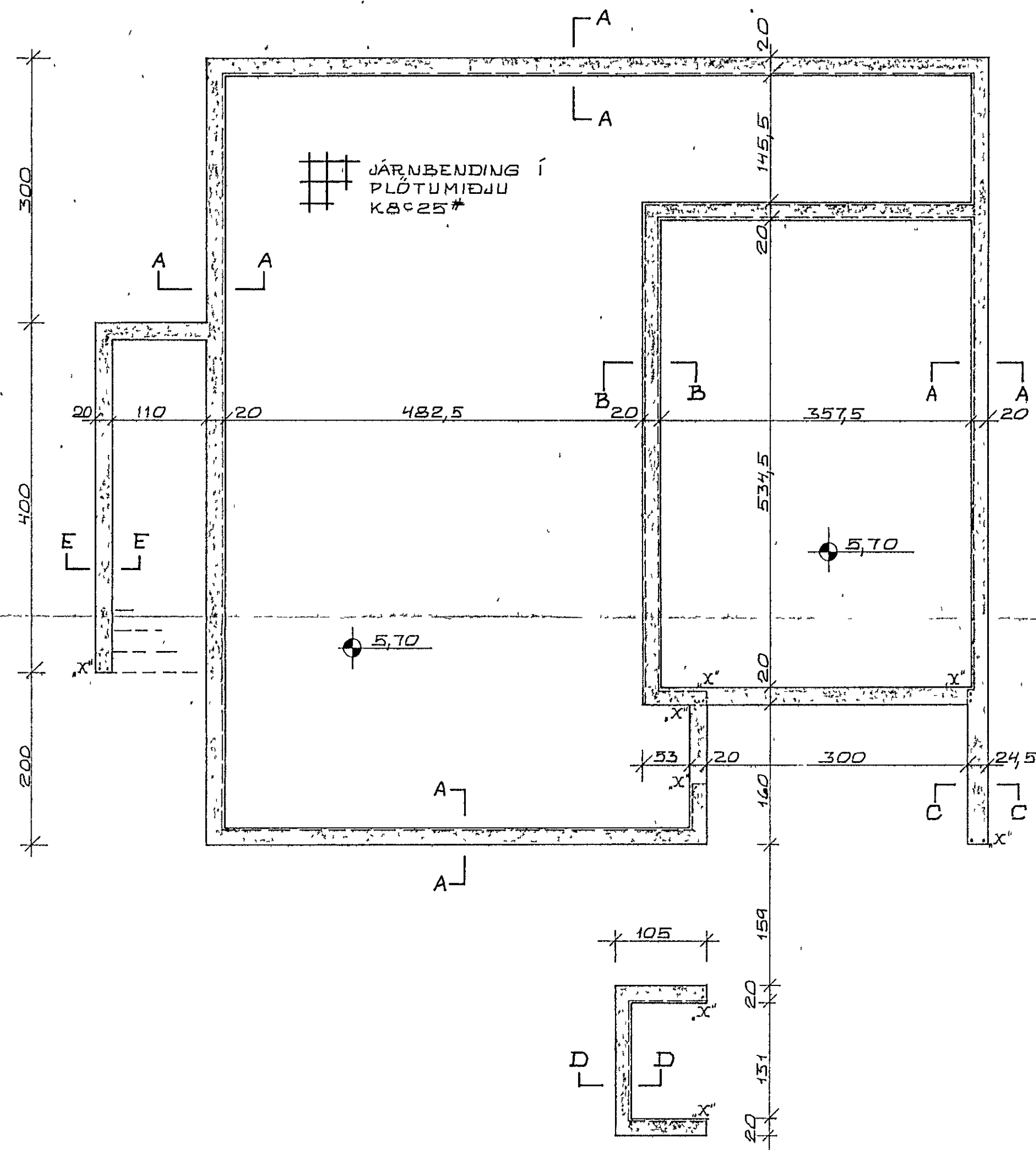
GRUNNMYND 1.50
