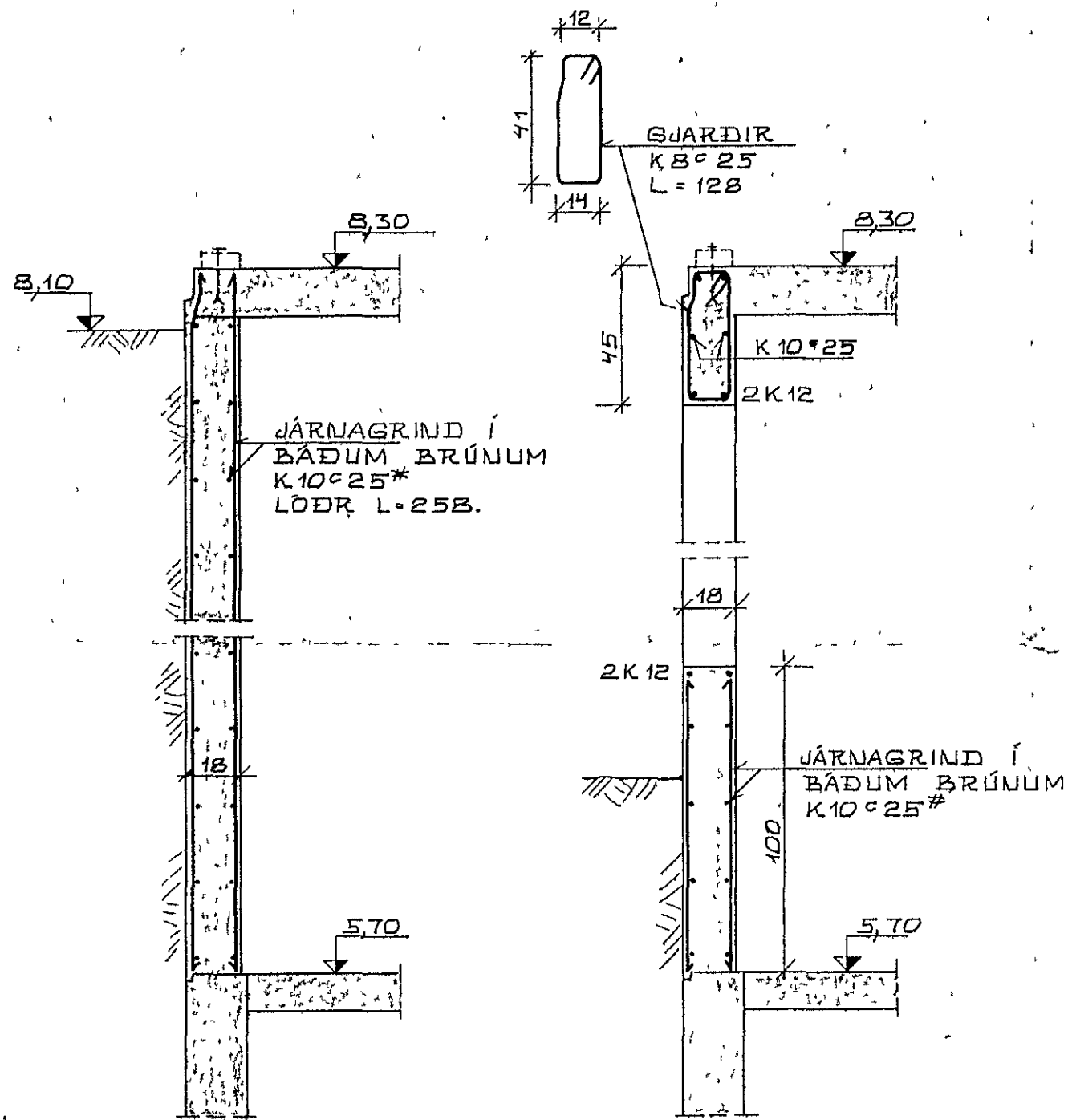
SNID 1-1 1:20
