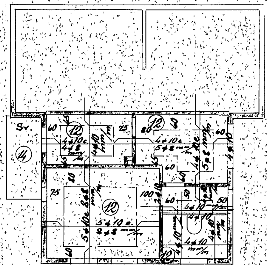
Loftr yfir kjallara 1:100
