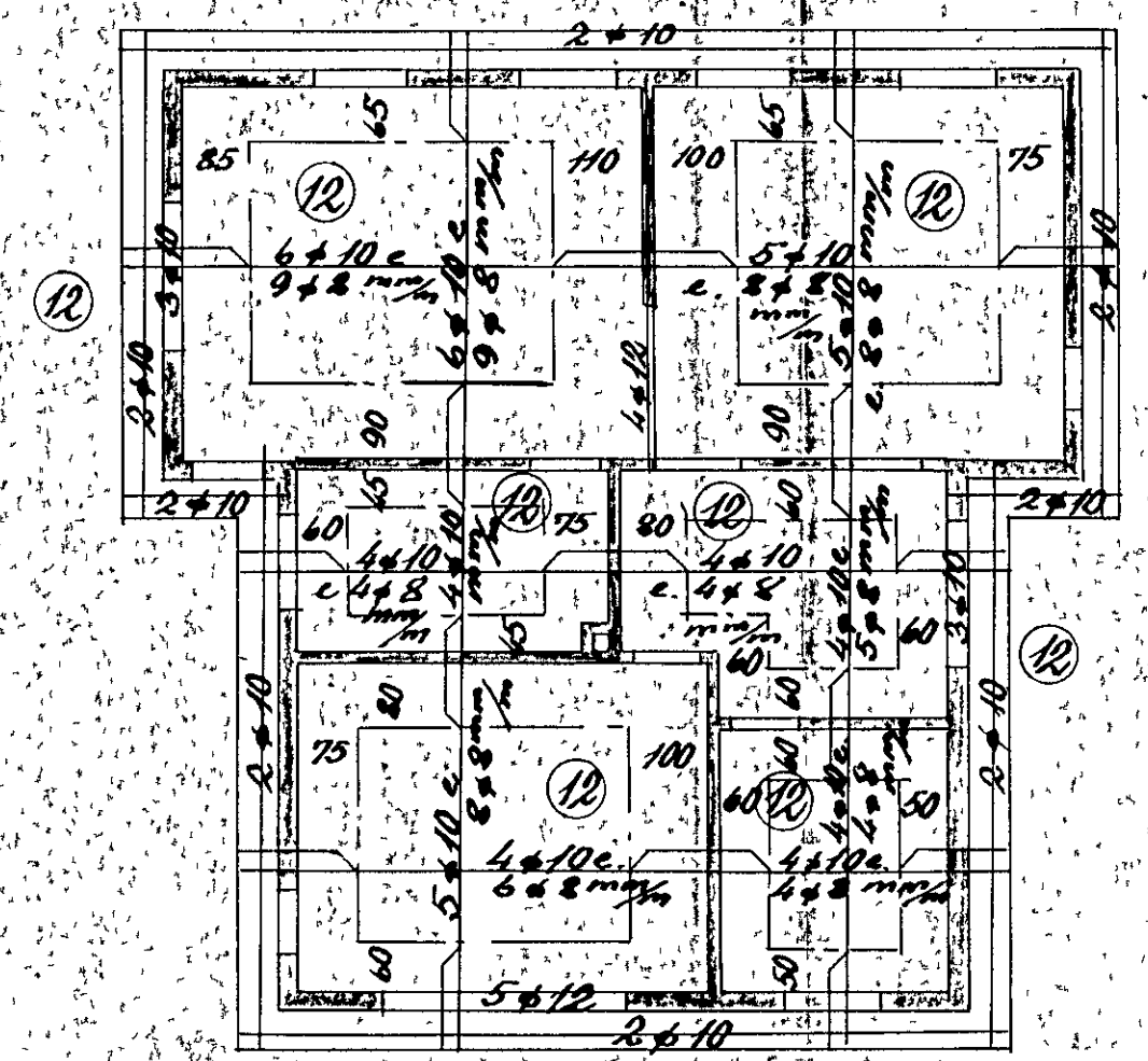
Loftr yfir hæð 1:100
