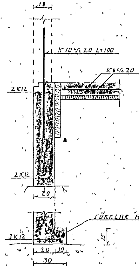
SNID A-A 1:20
