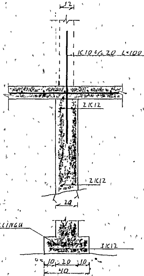
SNID B-B 1:20
