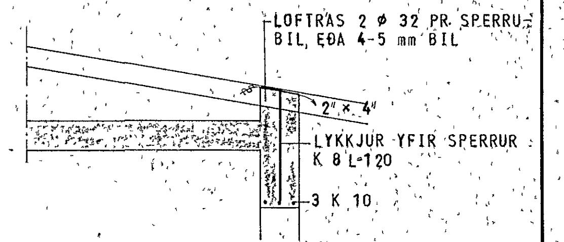
SNID E 1:20
