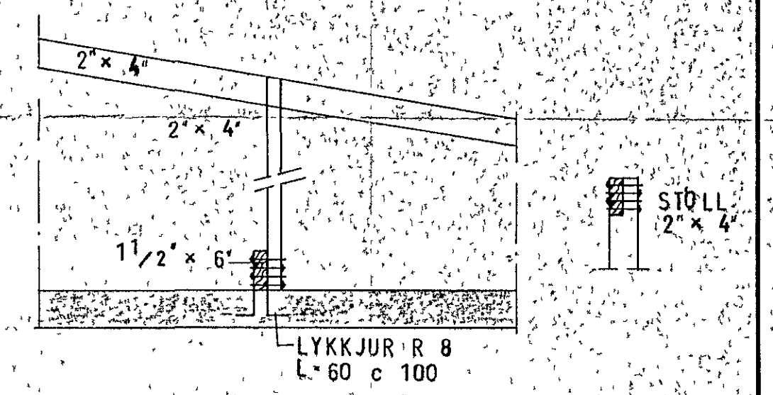
SNID D 1:20
