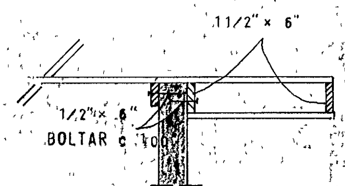
SNID G 1:20
