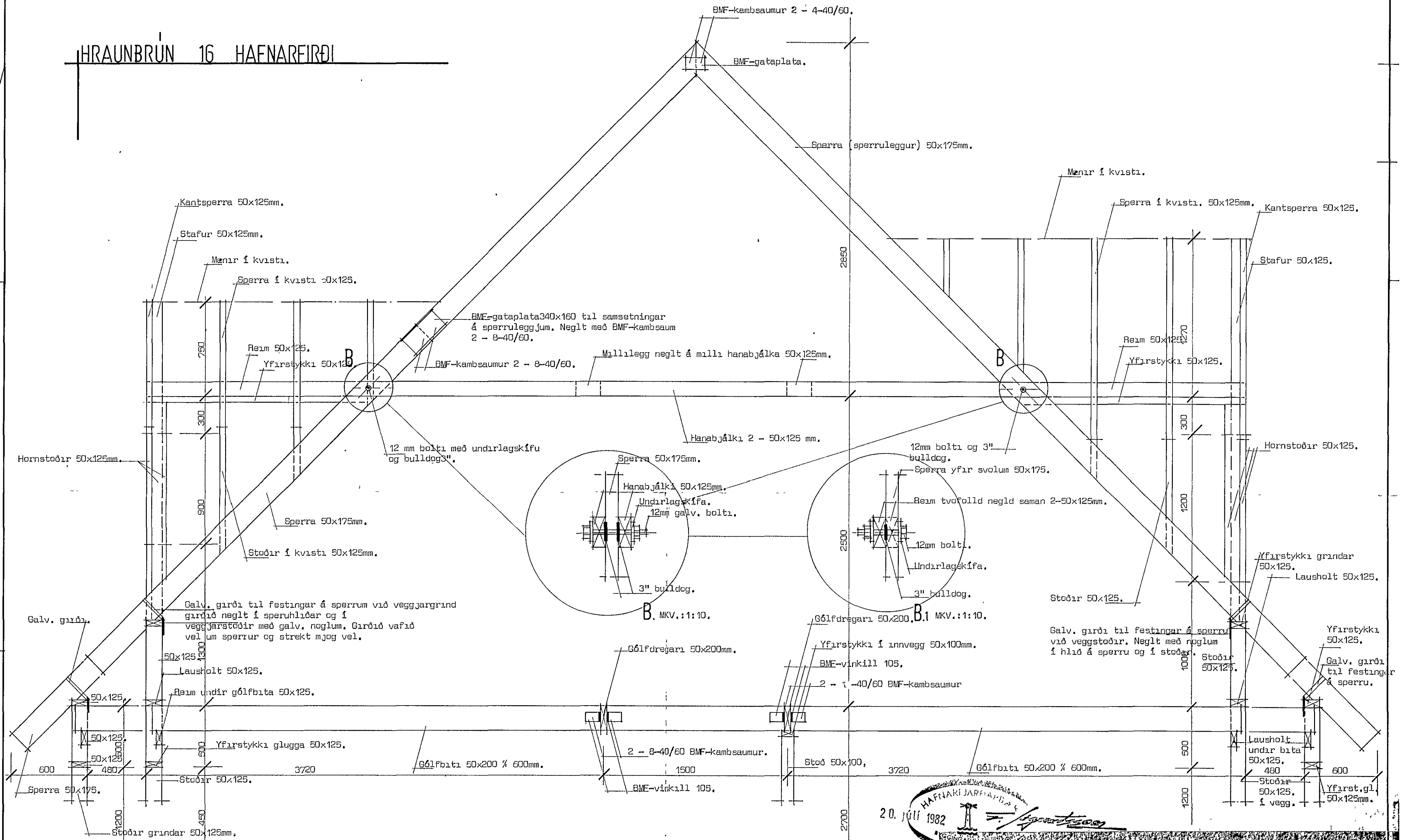
A-A, MKV.: 1:20.
