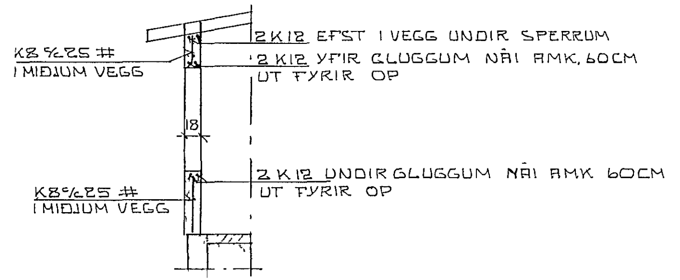
NORMALSNID 1:50
