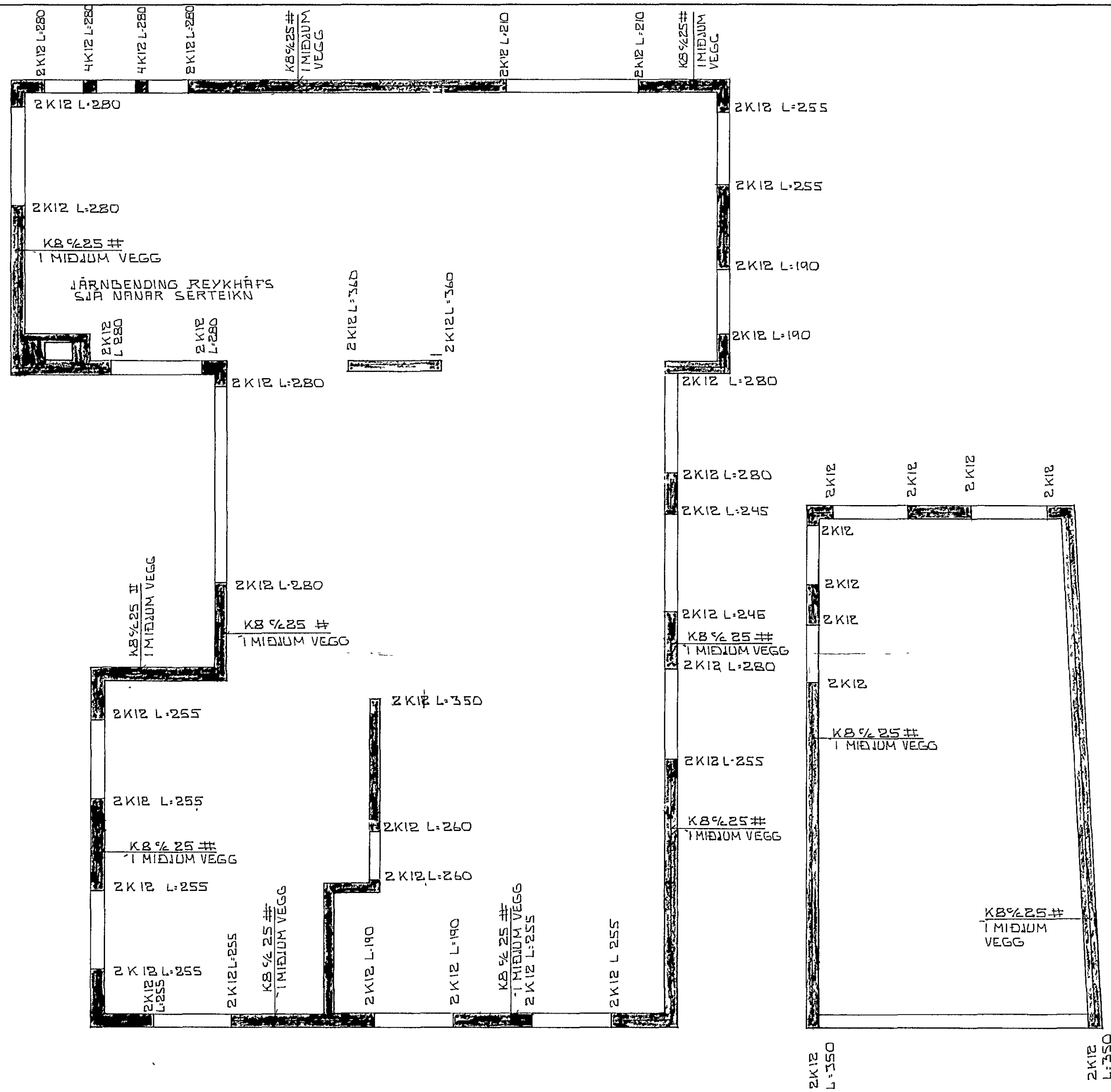
GRUNNMYND 1:50
