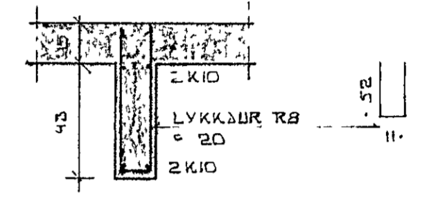
SNID B-B 1:20
