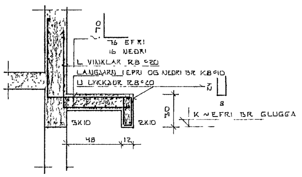
SNID A-A 1:20
