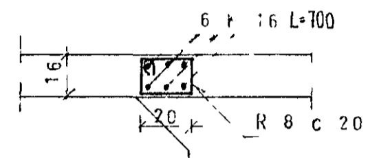
SNID D 1:20
