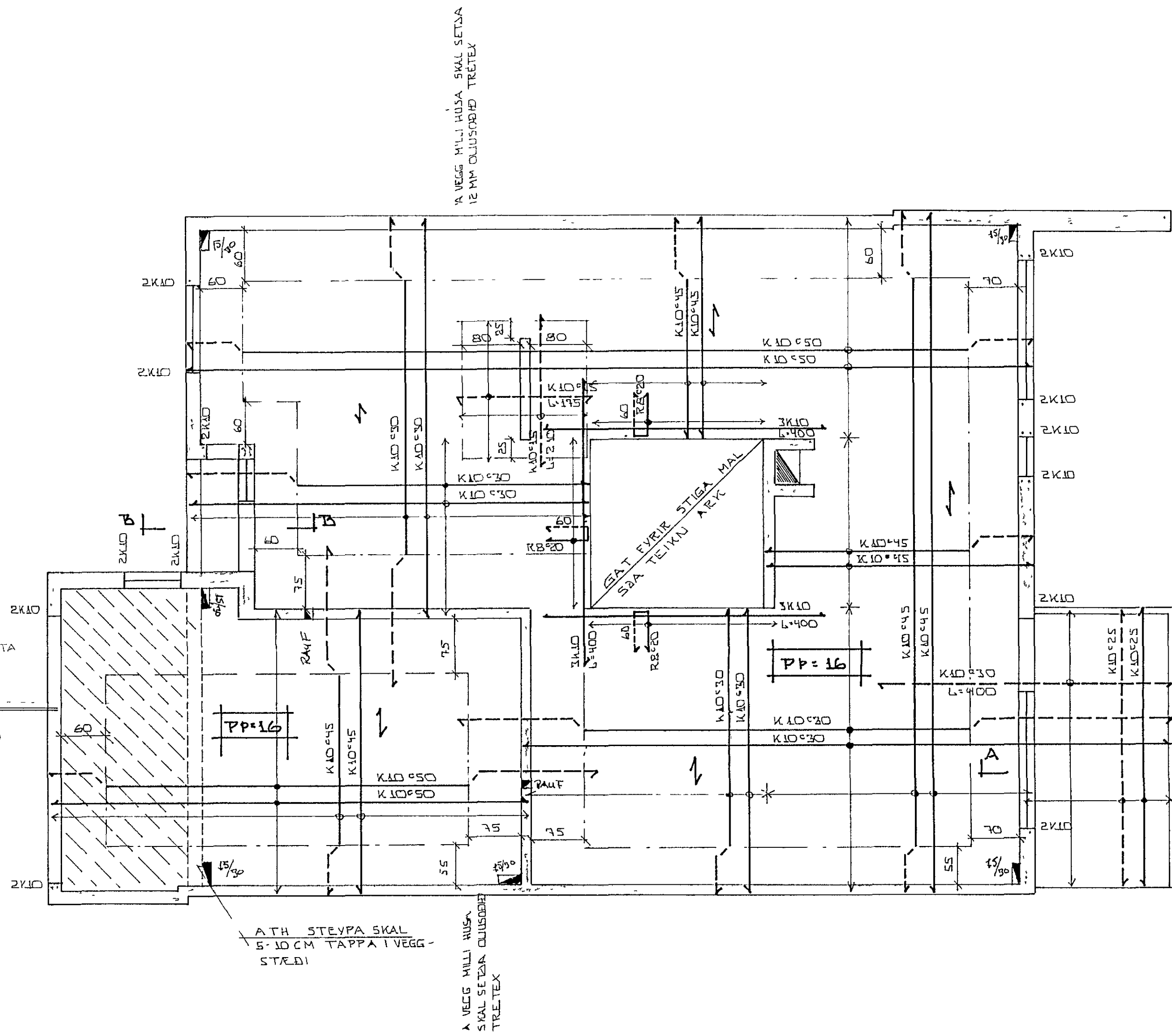
GRUNNMYND ~ 1:50
