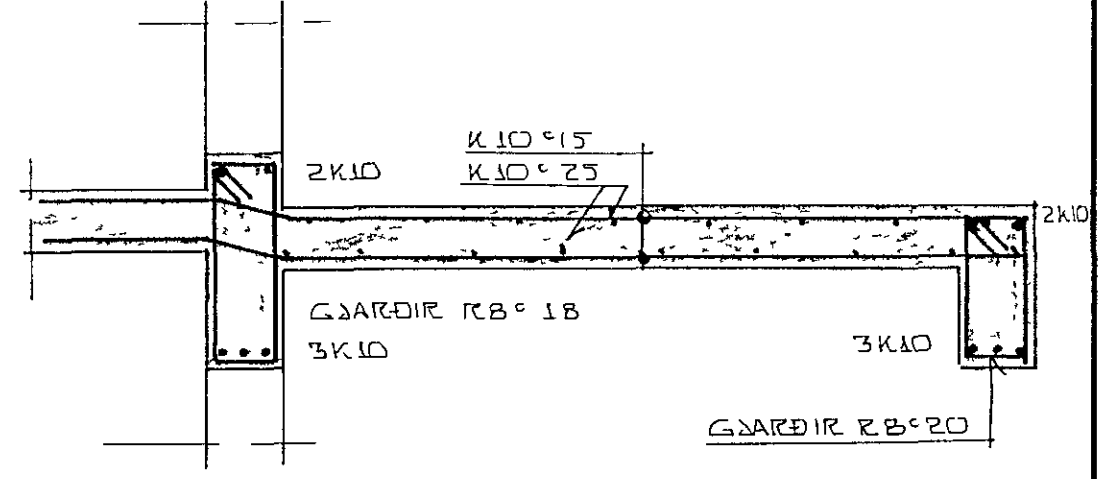
SNID A-A -1.20
