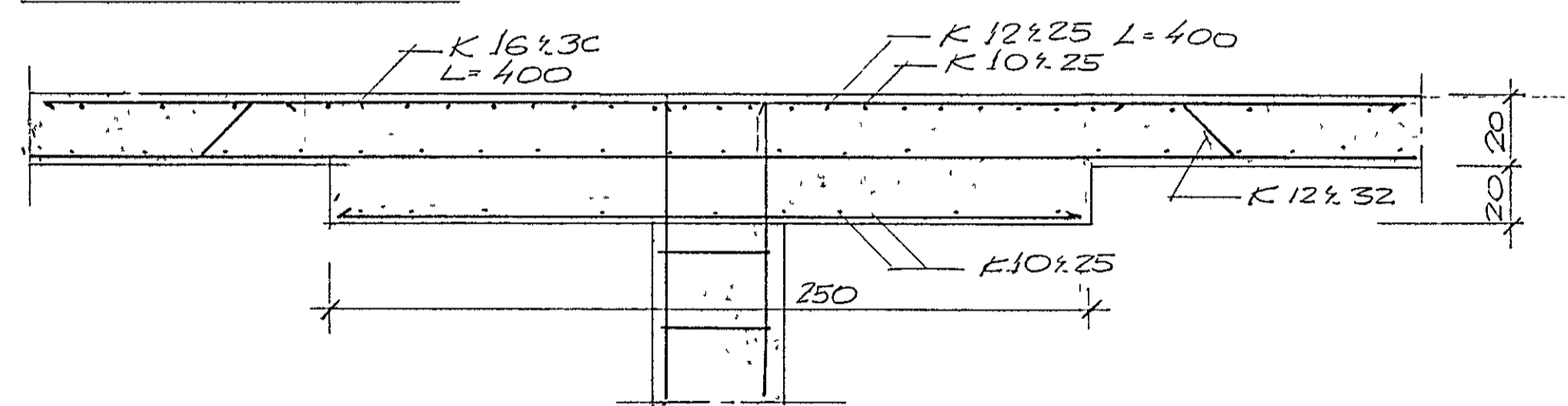
SNÍÐ E-E 120
