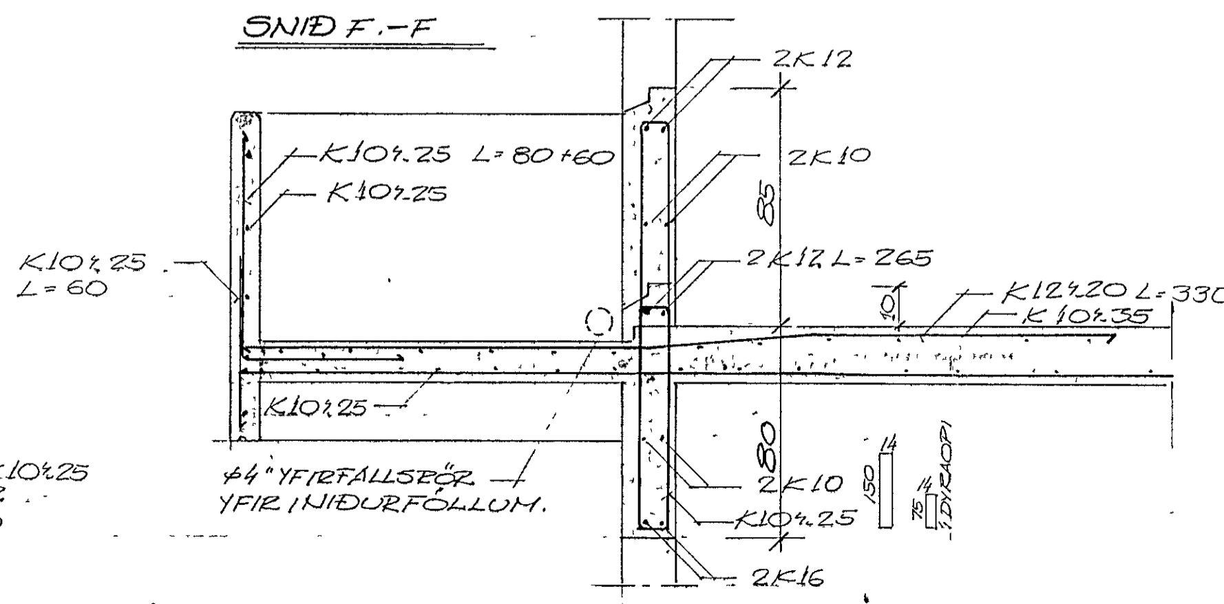
SNÍÐ F-F
