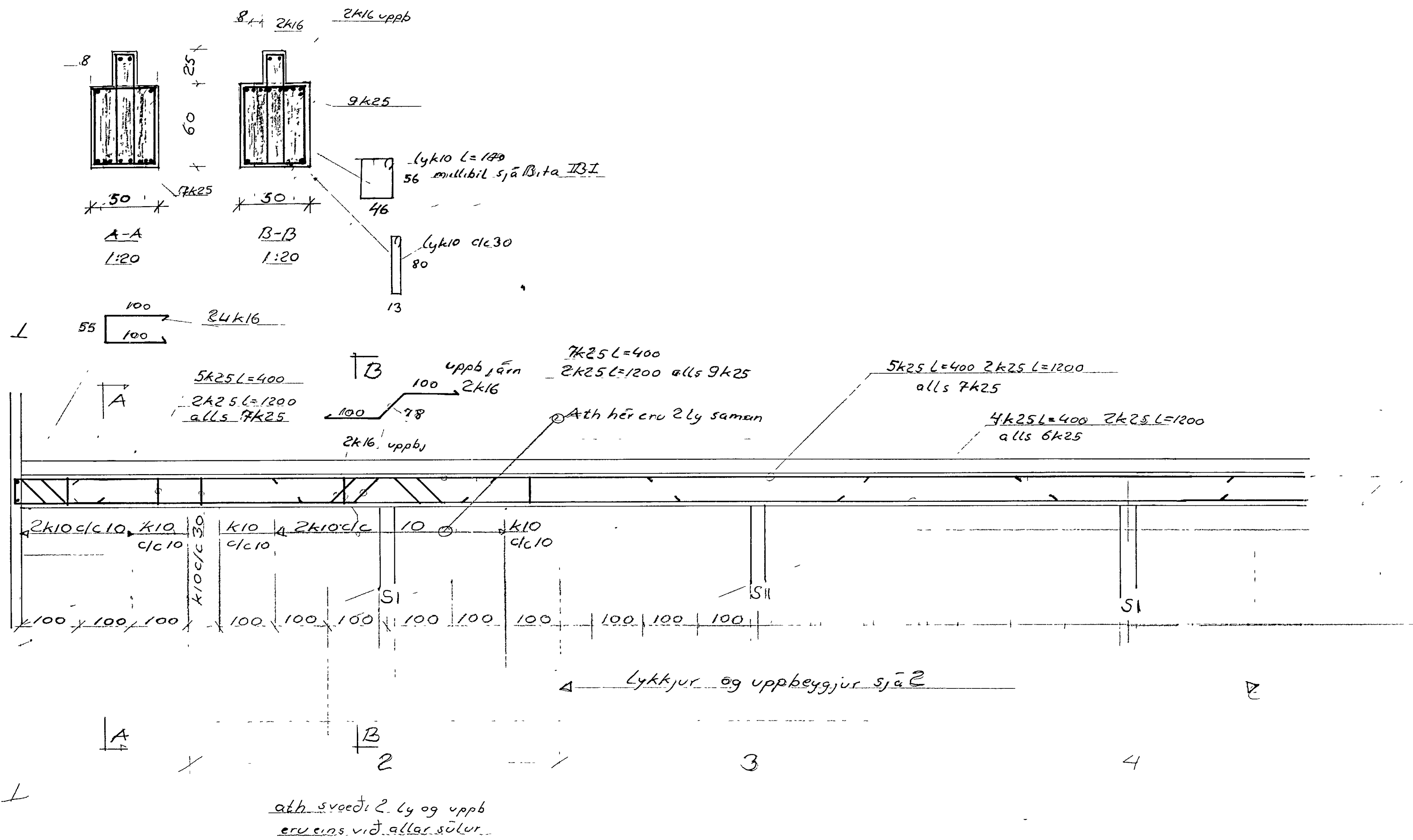
Beti B1 1:50
