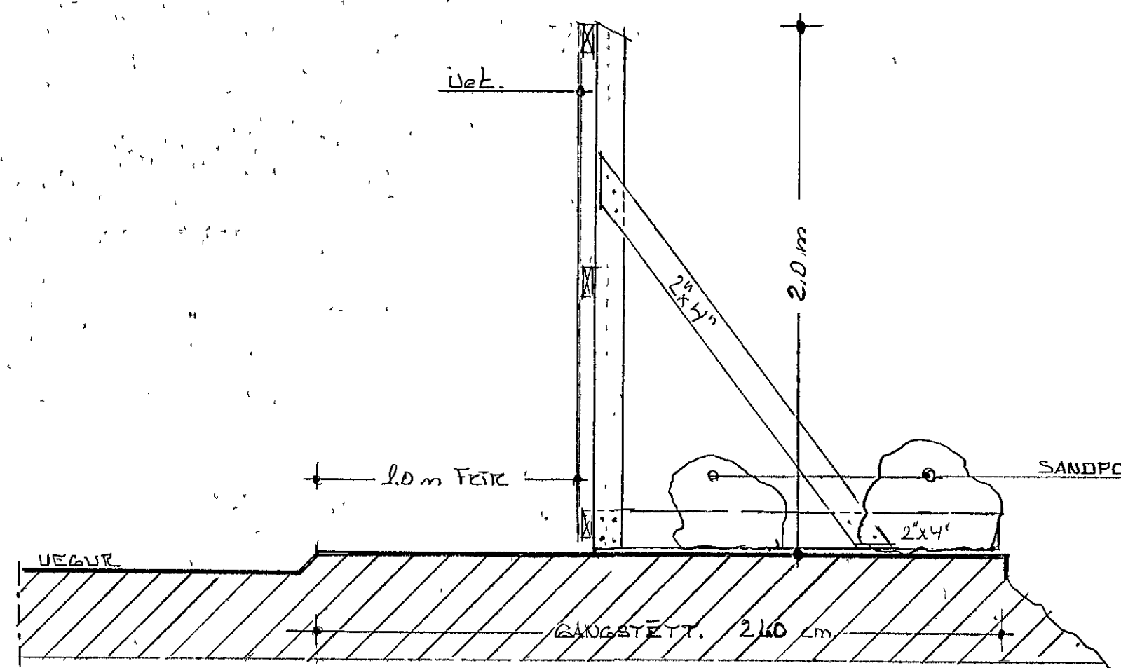
Snæðing í gangstétt þar sem girdingin stendur á henni. 1:20
