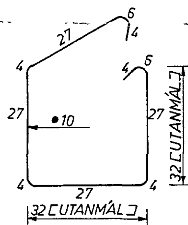
LYKKJUR L1 1:10
