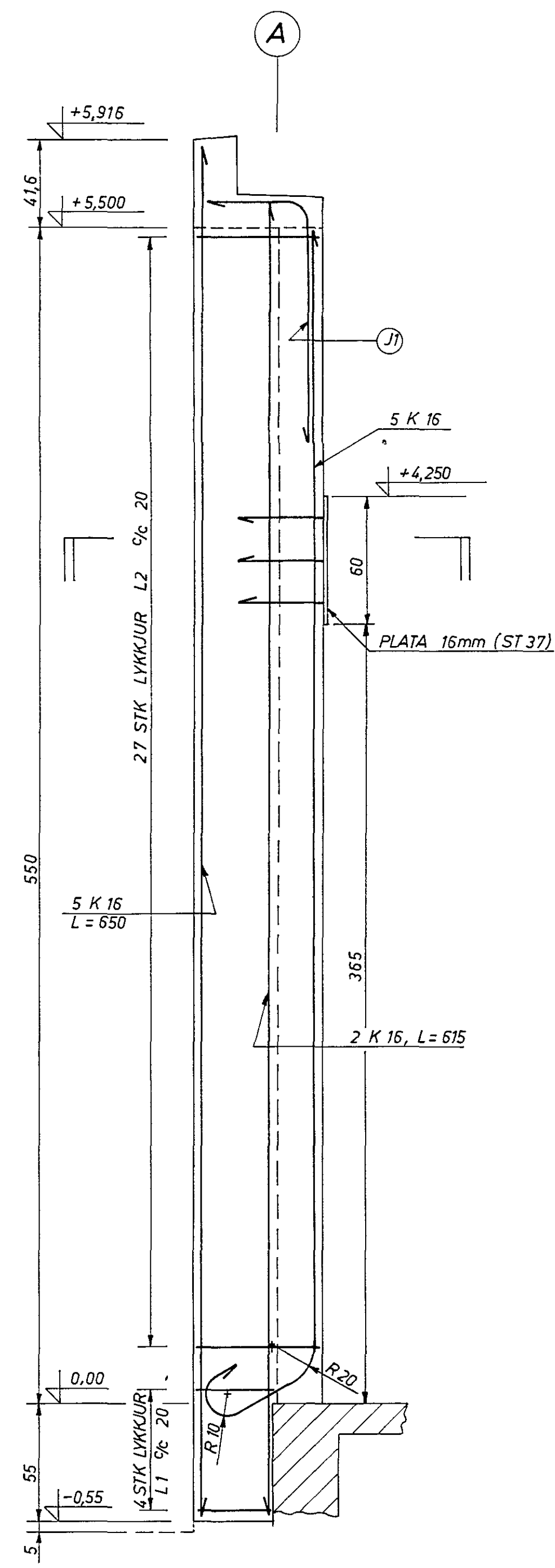
SÚLA 1:20
