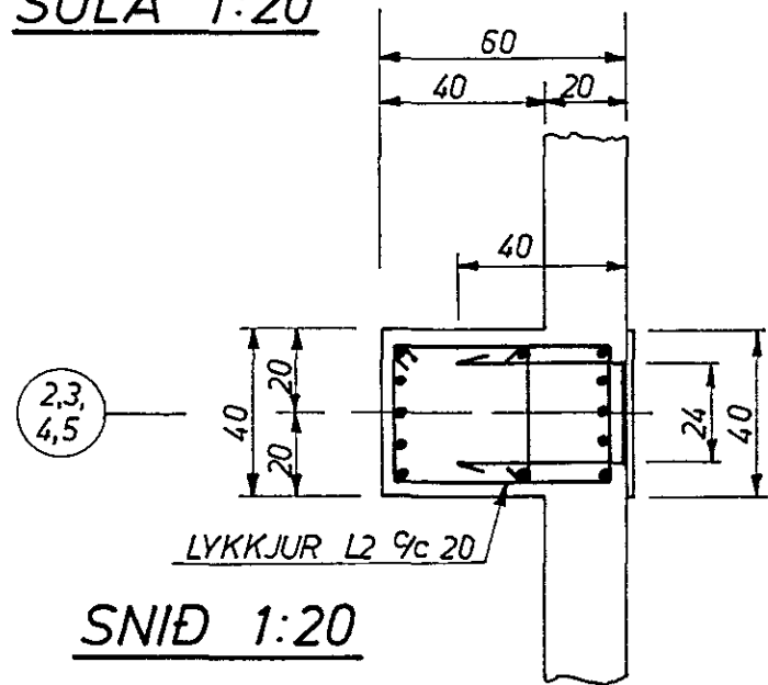
SÚLA 1:20
