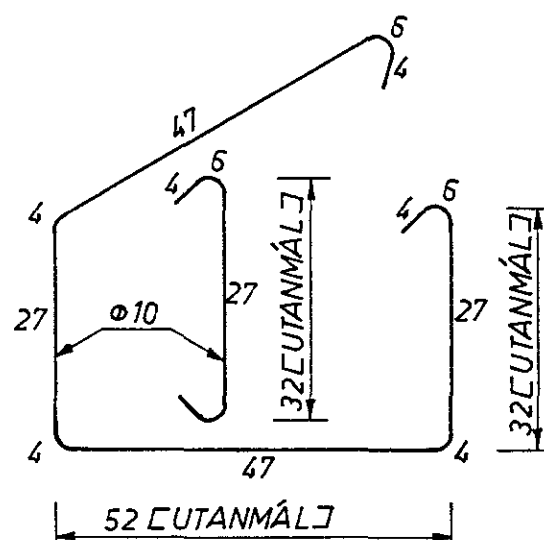
LYKKJUR L2 1:10
