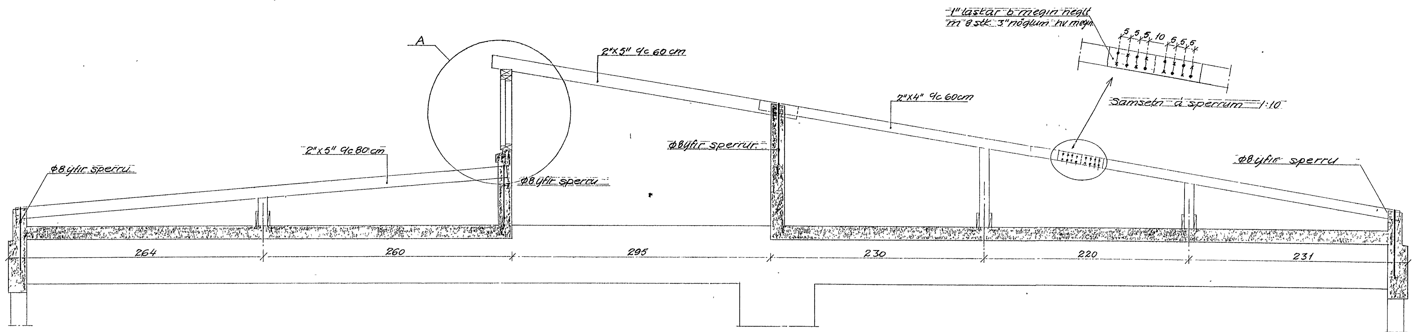
Þversnið 1:20
