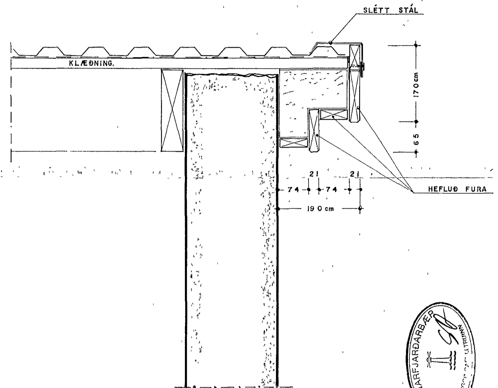
ÞAKKANTUR Á GAFLVEGGJUM. 1:5
