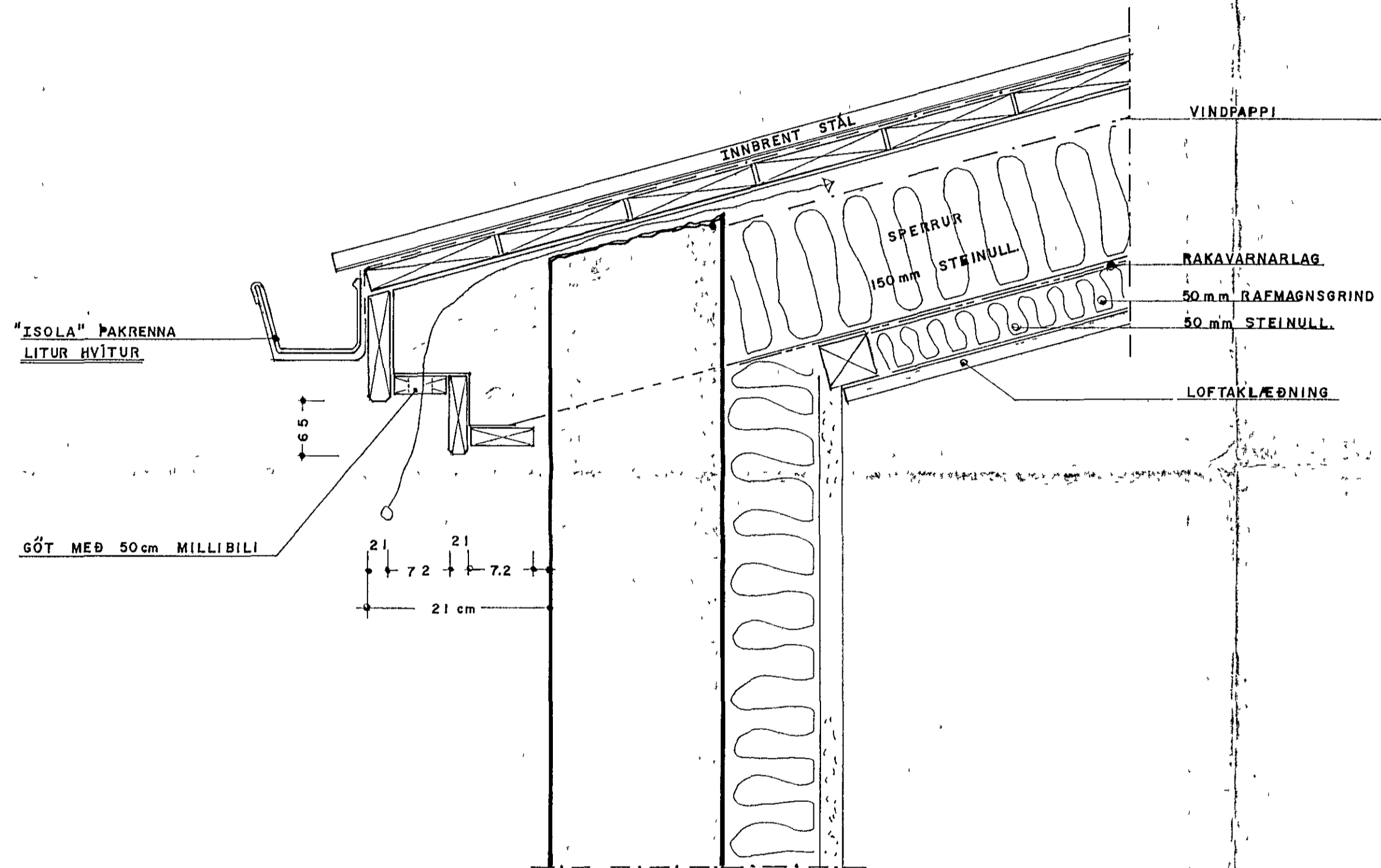
ÞAKKANTUR. 1:5
