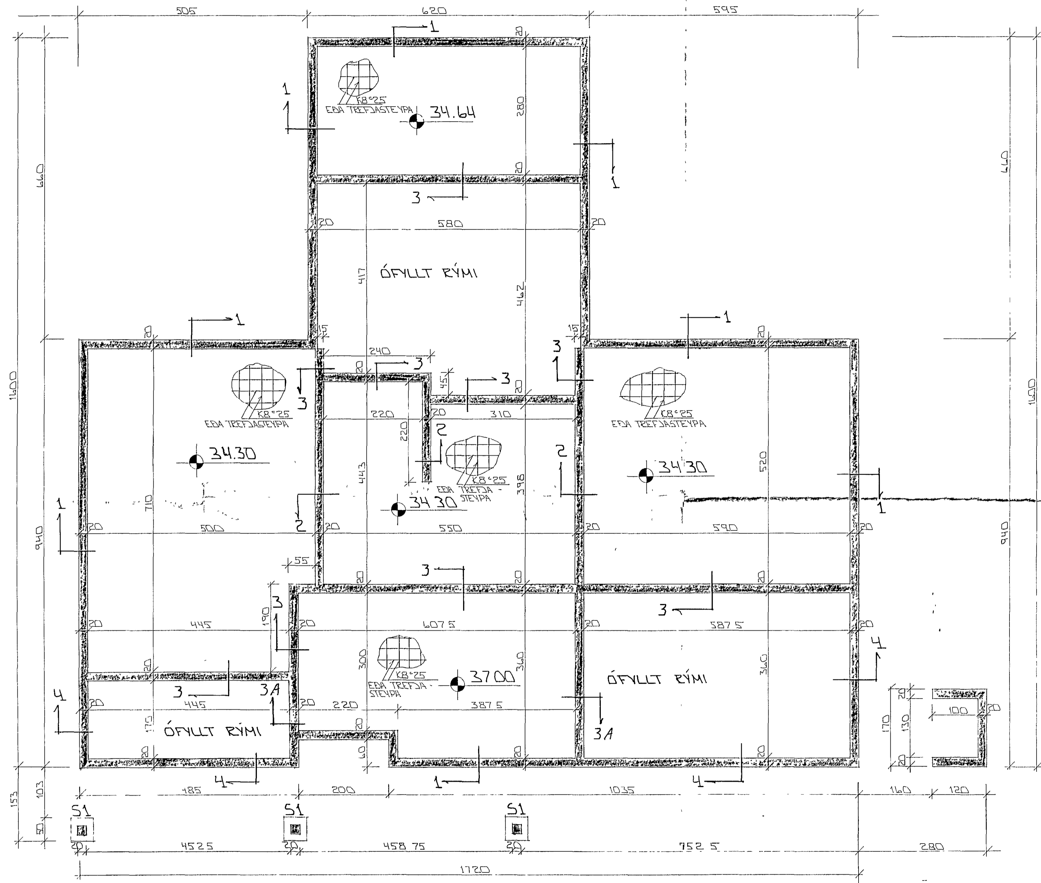
GRUNNMYND · 1:50
