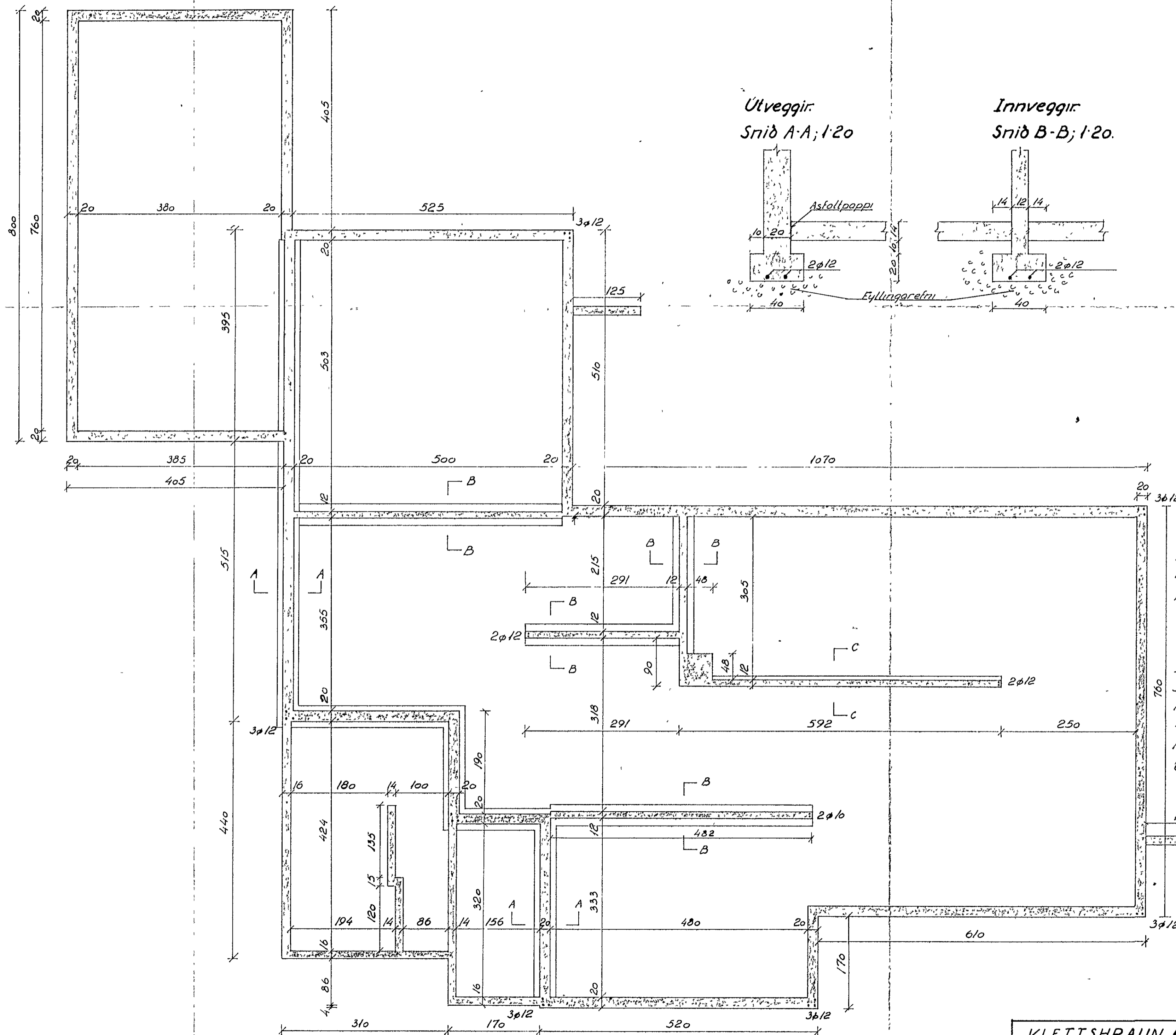
Grunnmynd, undirstöður, 1:50
