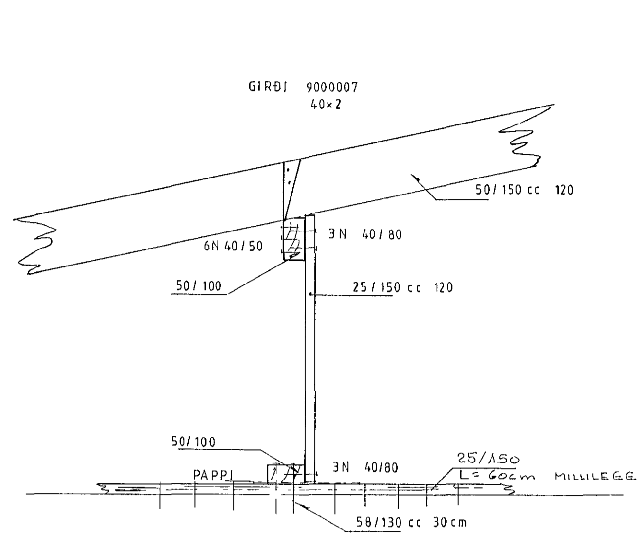
PAKSTÓLL 1 10
