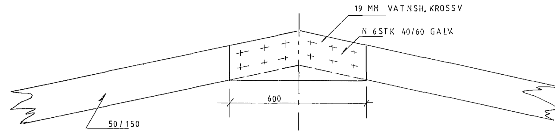
MÆNIR 1 10
