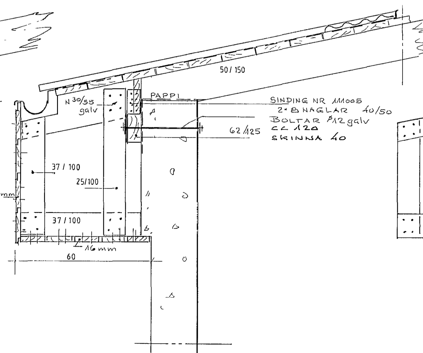
PAKBRÚN 1:10
