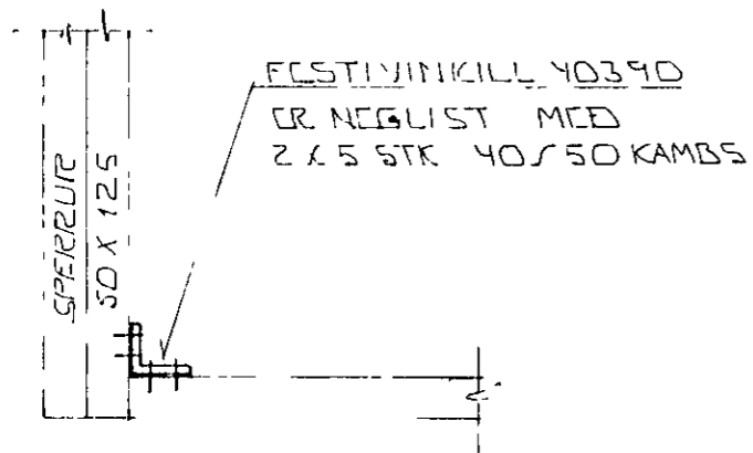
SERMYND 2 - 1:10
