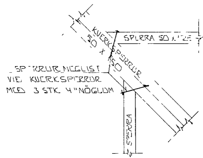
SERMYND 3 - 1:10
