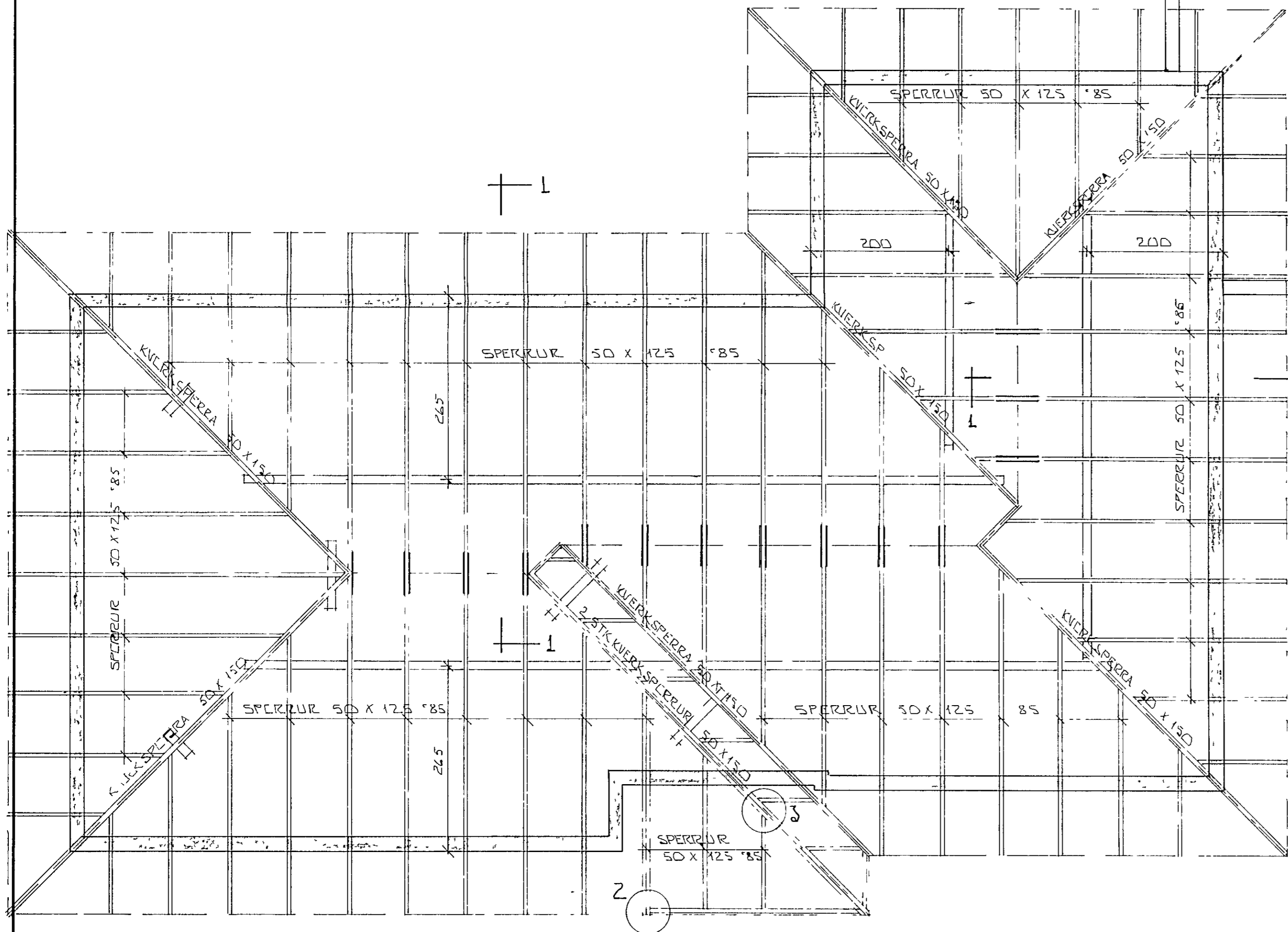
GRUNNMYND - 1:50
