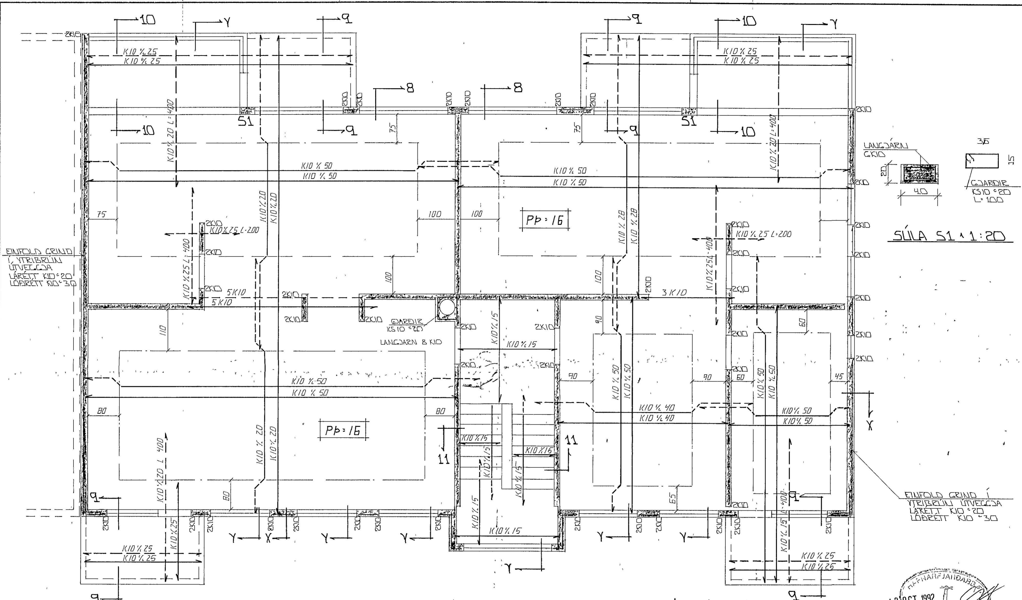
GRUNNMÝND · 1:20
