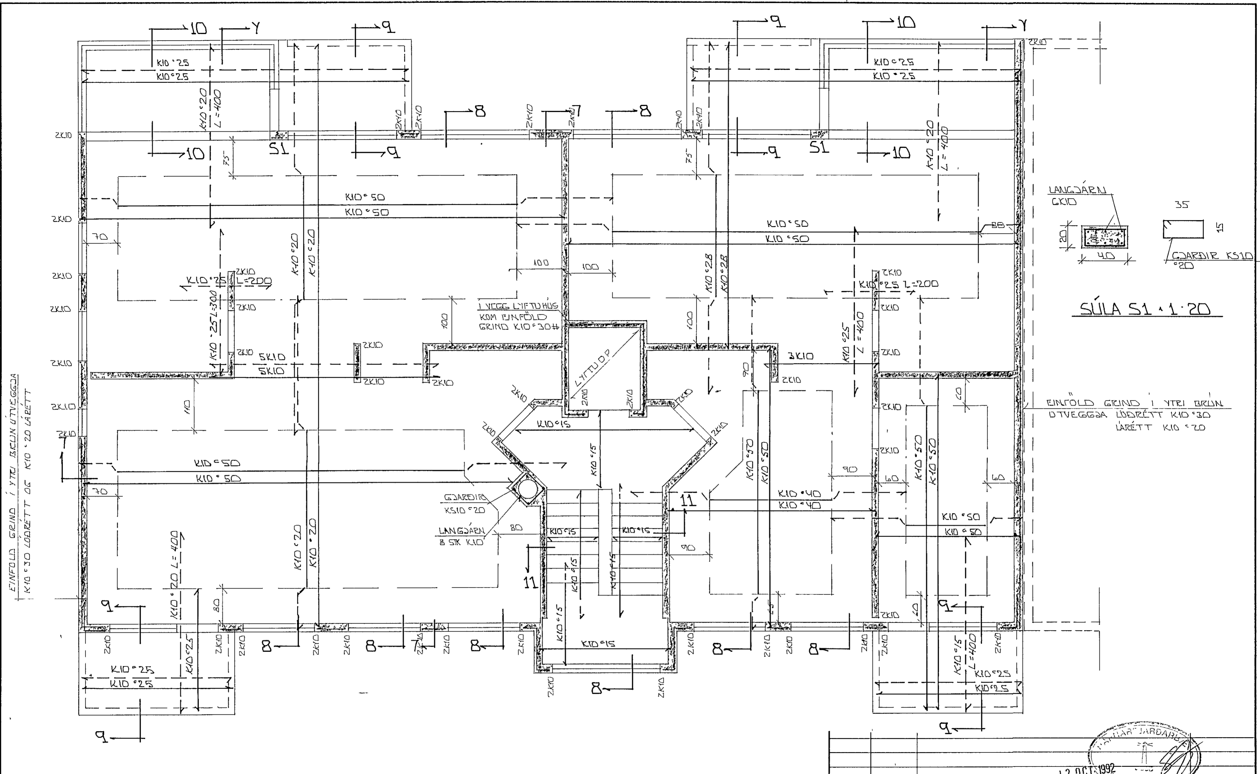
GRUNNMÝND · 1 · 50
