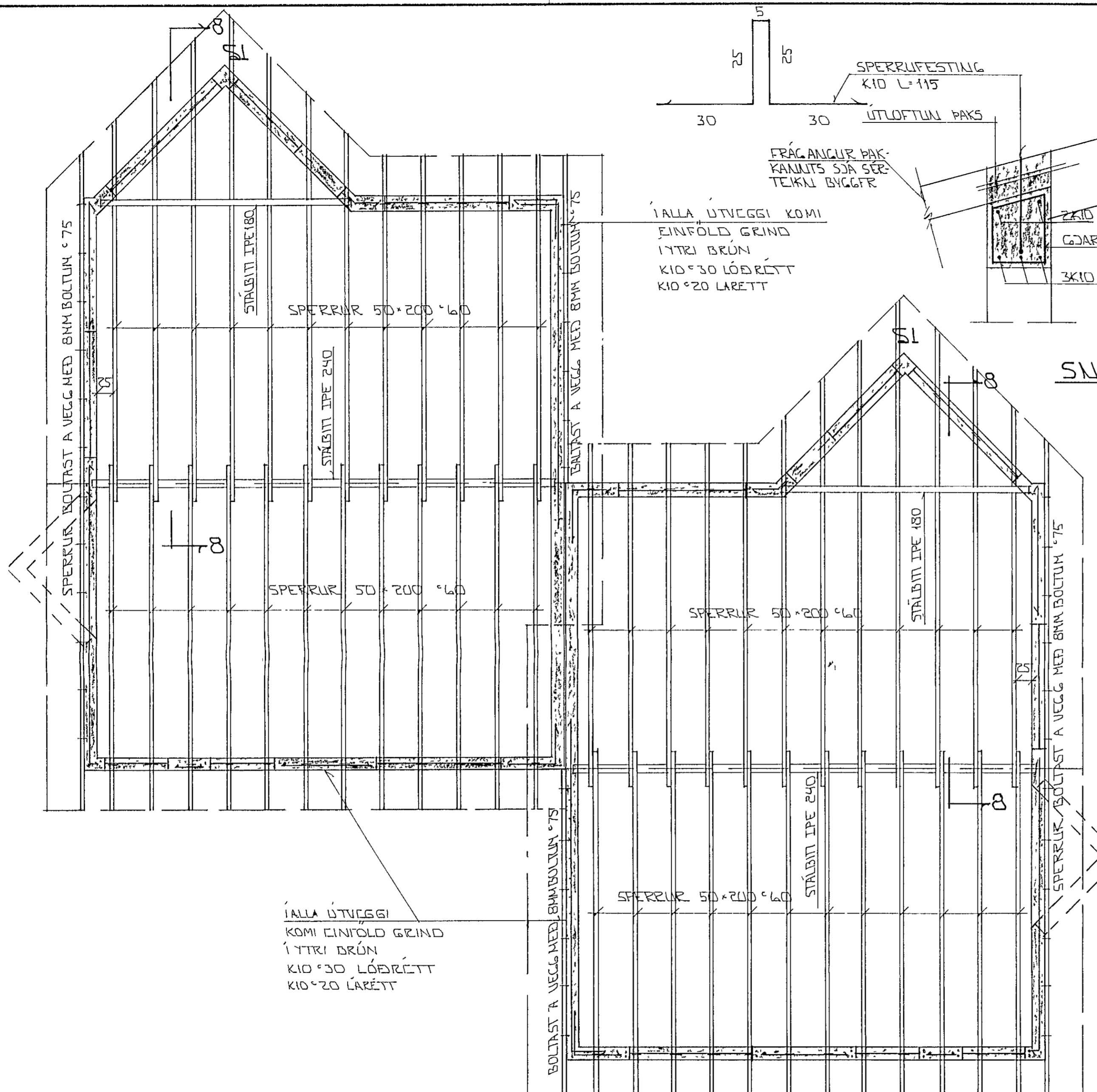
GRUNNMÝND ÞAKS 1:50
