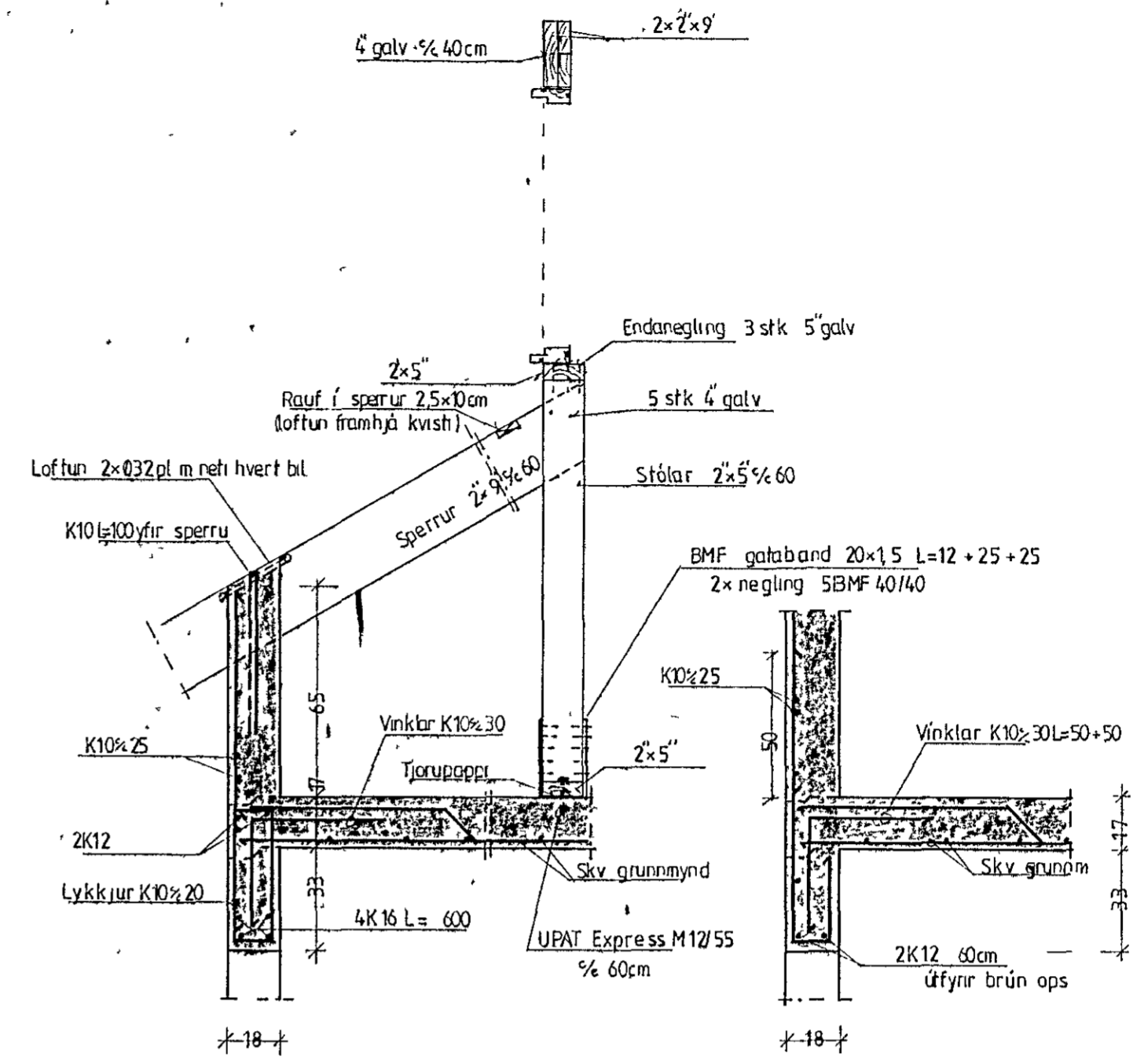
Snið P1 1:20
