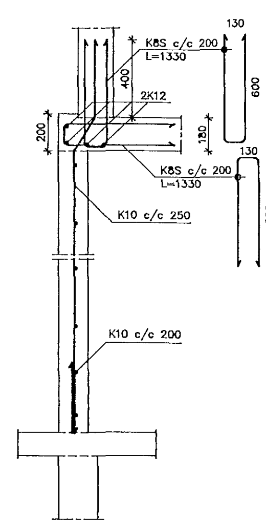
Snið K06 1 20
