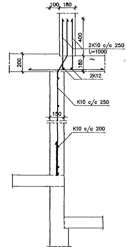
Snið J06 1 20
