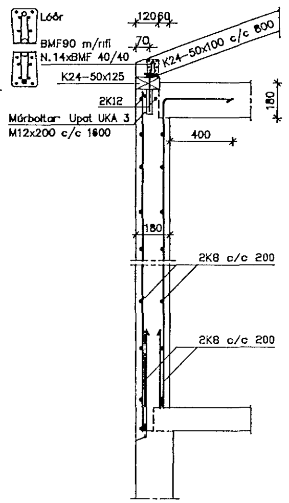
Snið D06 1 20
