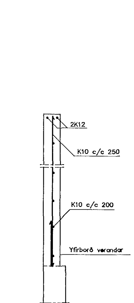
Snið N06 1 20
