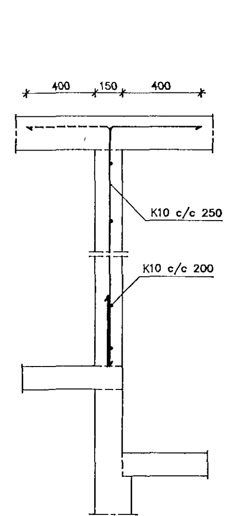
Snið I06 1 20
