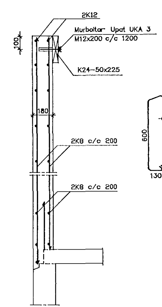
Snið A06 1 20
