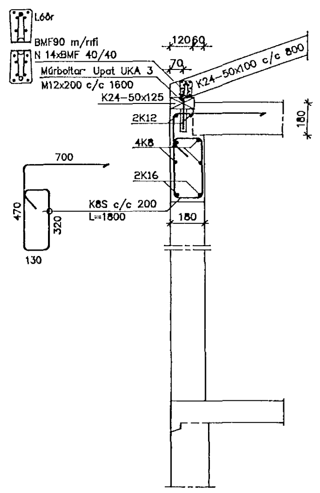
Snið G06 1 20
