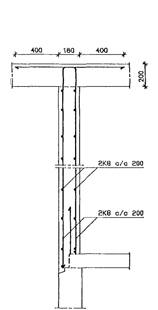
Snið H06 1 20
