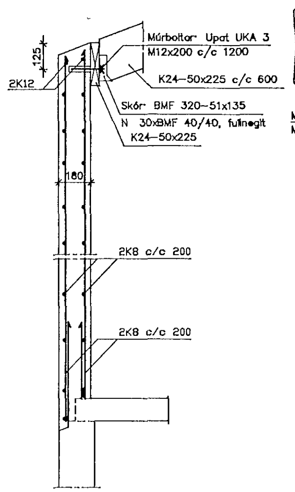
Snið C06 1 20
