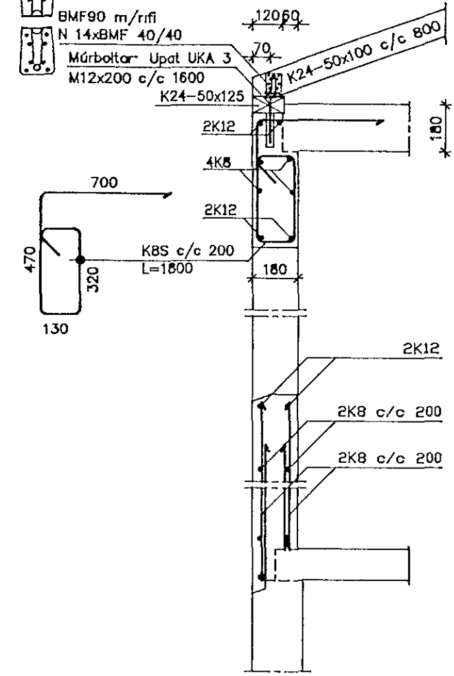
Snið E06 1 20
