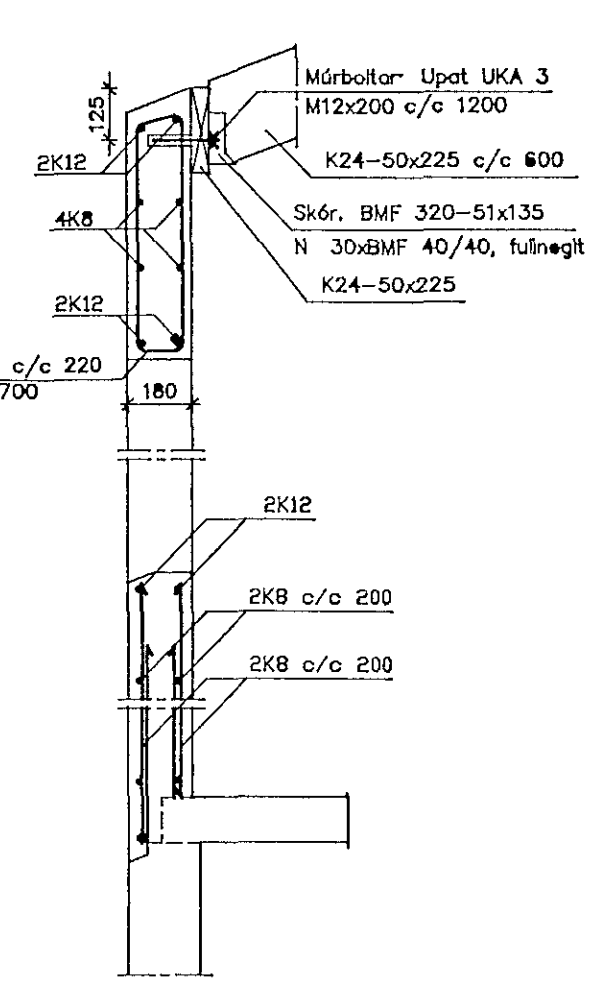
Snið B06 1 20
