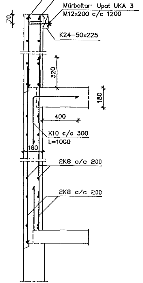
Snið F06 1 20
