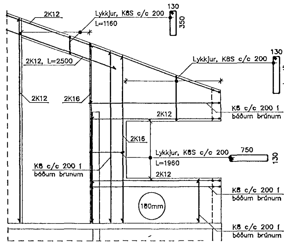
Snið A07 1 : 50
