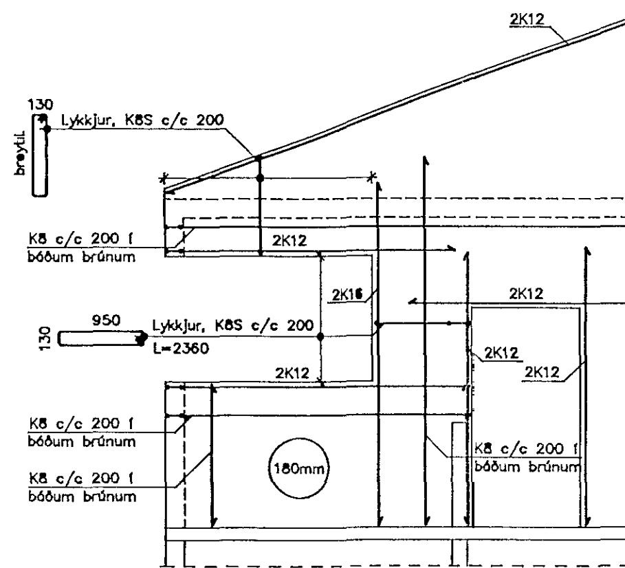
Snið B07 1 : 50
