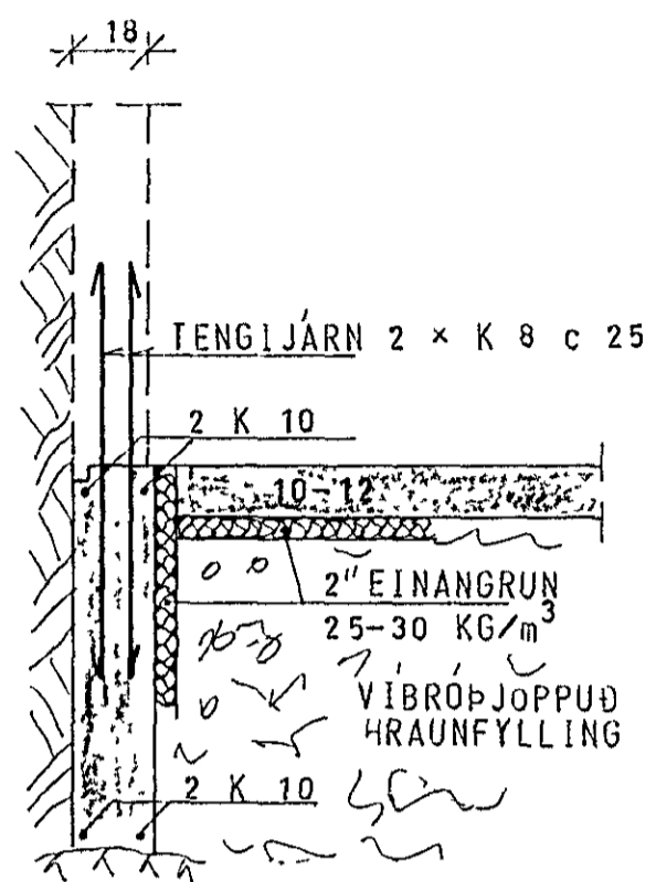
SNIÐ Í ÚTVEGGI 1:20
