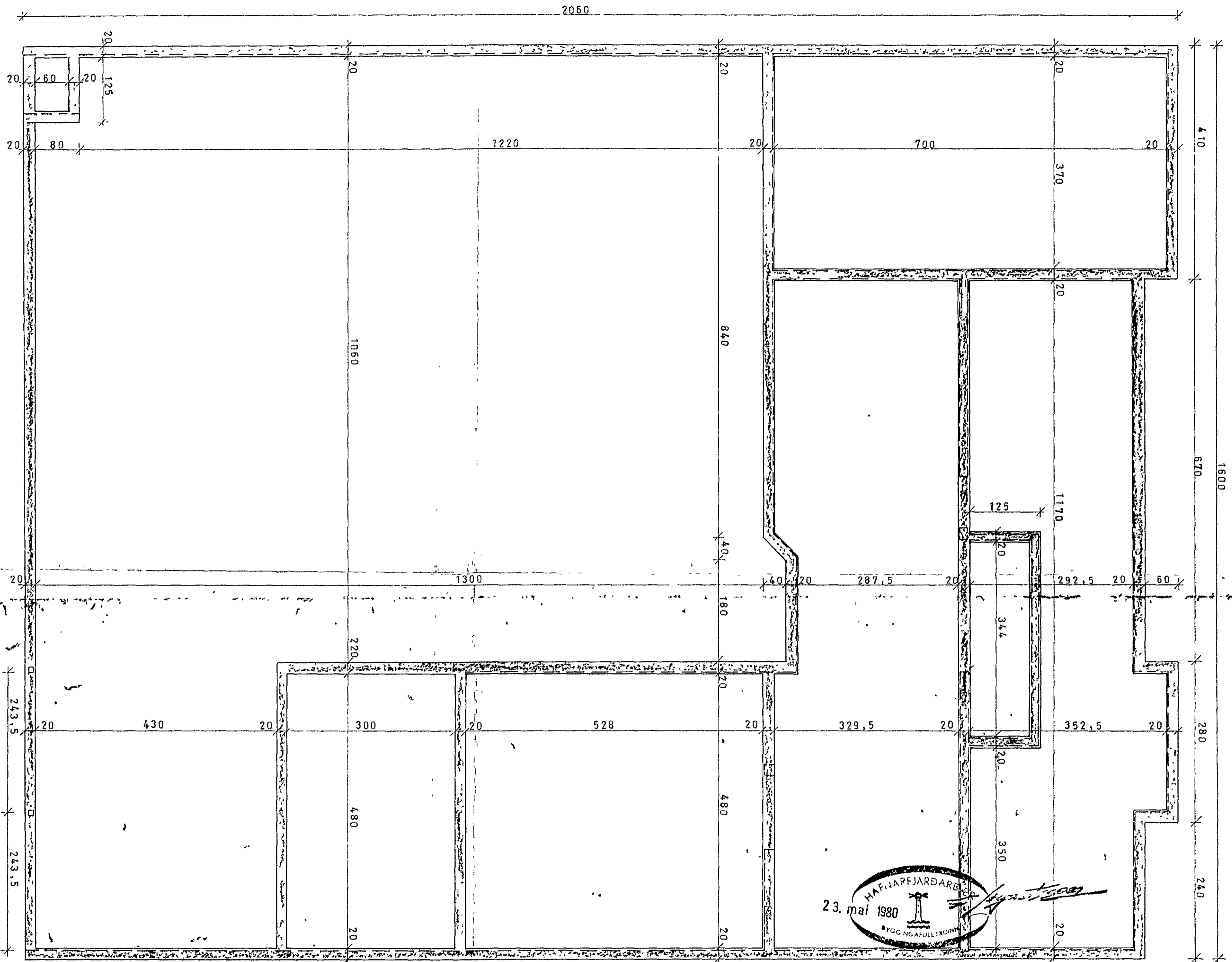
SNIÐ Í INNVEGGI 1:20
